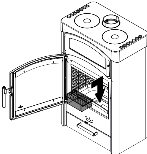
Abb. 31: Aschebox in Kaminofen einbringen
