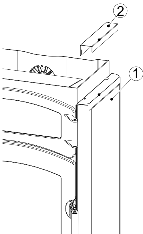
Abb. 15: Specksteinseitenverkleidung einhängen
