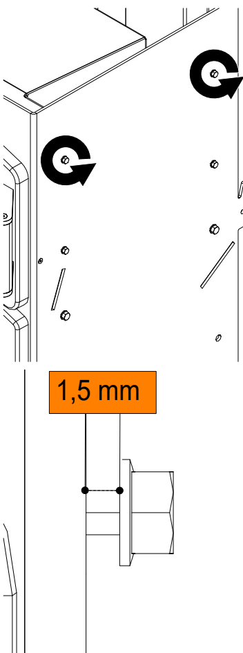
Abb. 14: Schrauben aufdrehen
