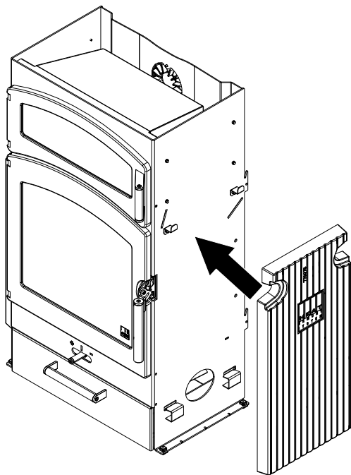
Abb. 18: HMS-Stein anbringen
