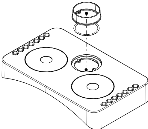
Abb. 24: Stützen und Dichtung vom Deckel demontieren
