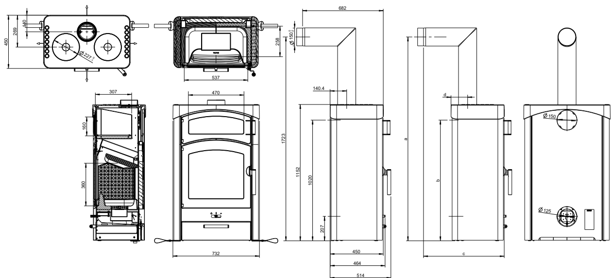
Abb. 2: Abmessungen
