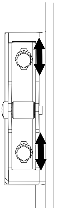
Abb. 34: Türverschluss einstellen
