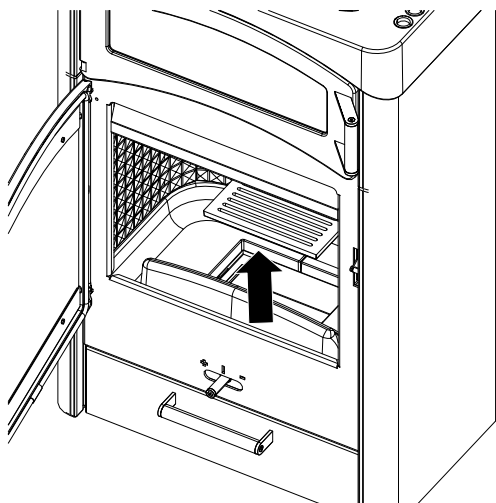
Abb. 39: Rost herausnehmen
