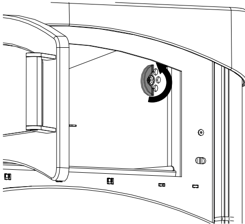
Abb. 35: Luftregler
