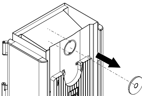
Abb. 25: Abdeckung demontieren
