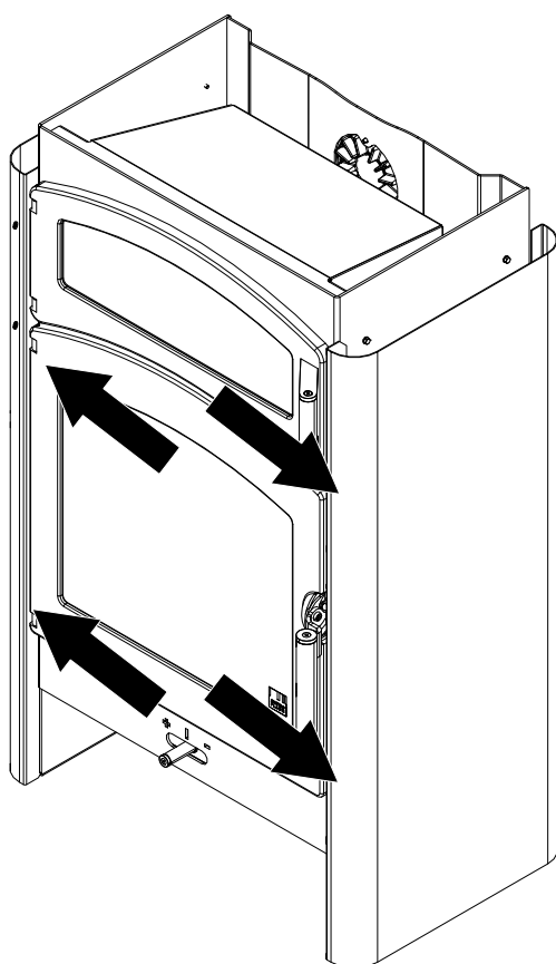
Abb. 46: Vordere vier Schrauben entfernen
