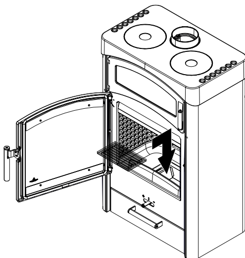
Abb. 33: Rost Aschebox einlegen
