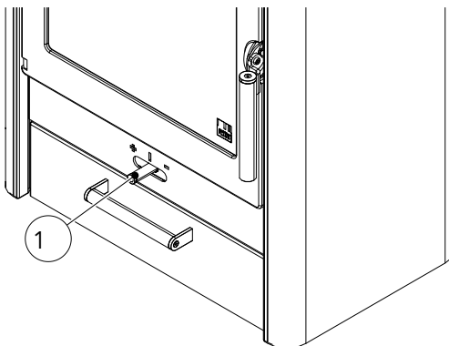
Abb. 36: Primär- Sekundärluftregler
