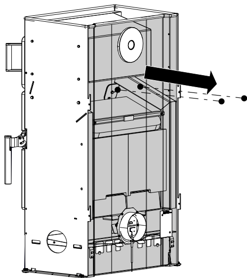
Abb. 16: Schutzblech entfernen
