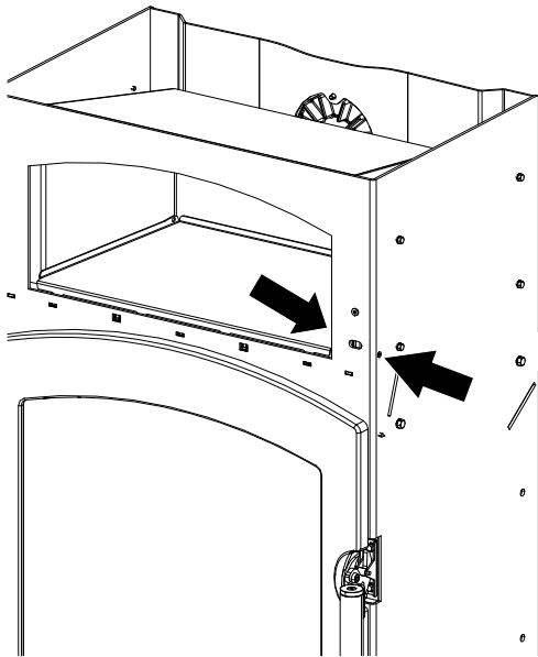
Abb. 9: Vormontierte Schrauben entfernen
