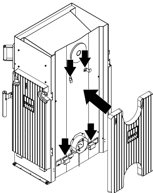
Abb. 20: HMS-Stein hinten anbringen
