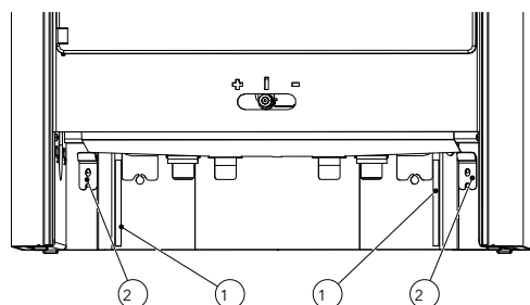
Abb. 30: Holzlade montieren
