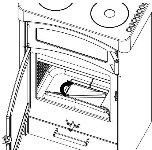
Abb. 40: Deckel auf Aschebox geben
