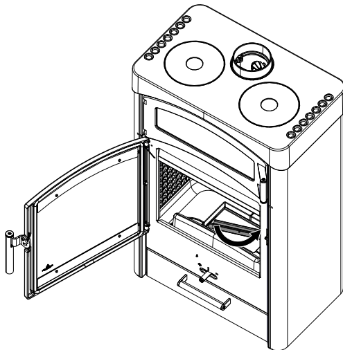
Abb. 32: Deckel Aschebox entriegeln
