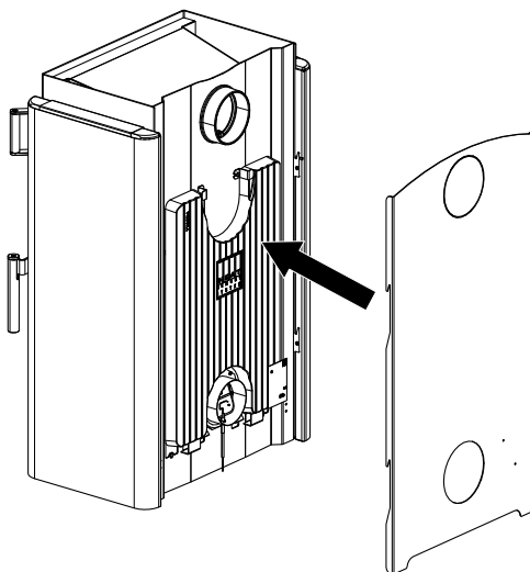
Abb. 27: Rückwand einhängen
