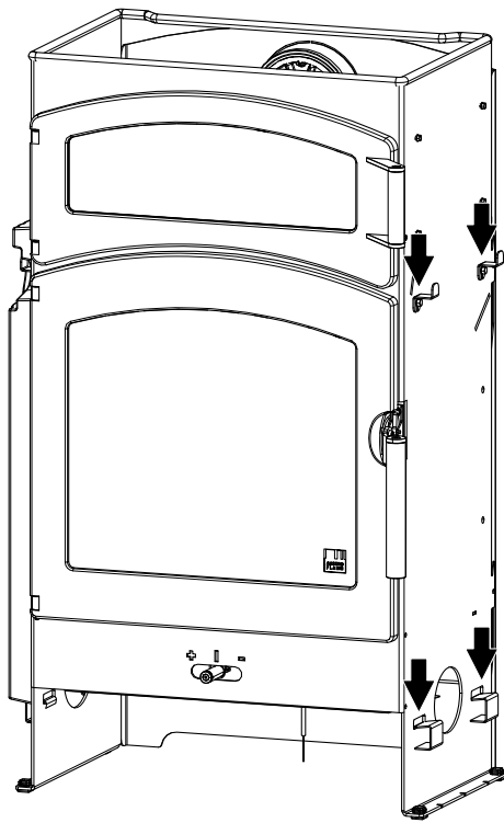
Abb. 17: HMS-Halter einhängen
