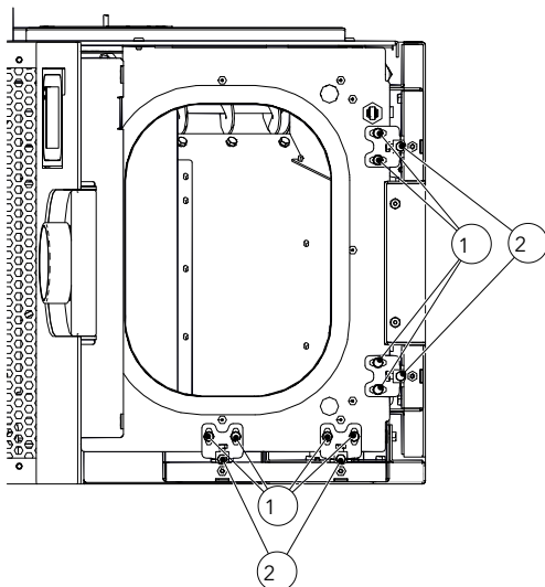
Abb. 15: Verkleidung einstellen
