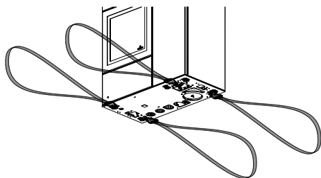
Abb. 7: Transporthilfe
