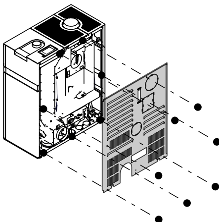
Abb. 26: Rückwand demontieren
