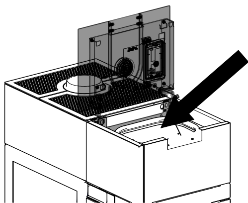
Abb. 44: Pellets füllen
