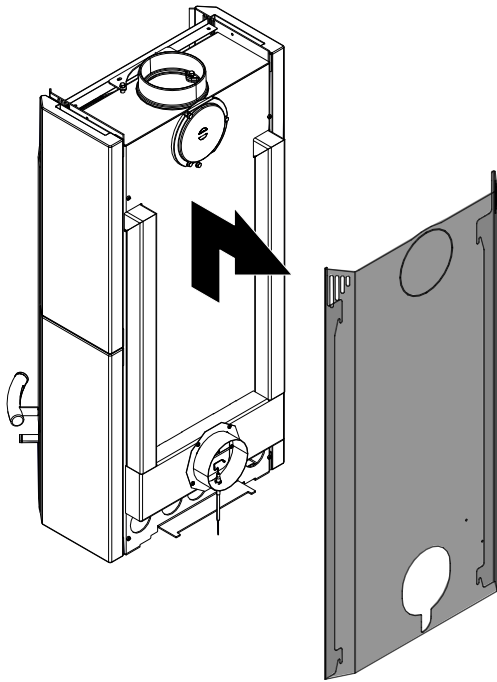
Abb. 19: Rückwand abnehmen
