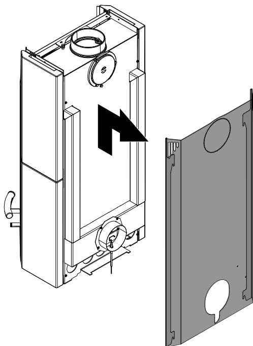
Abb. 52: Rückwand abnehmen
