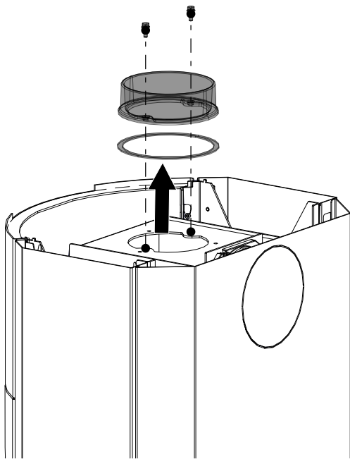
Abb. 20: Rauchrohrstutzen abmontieren
