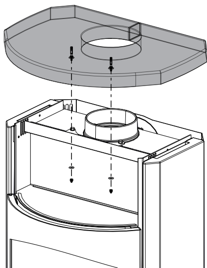
Abb. 18: Deckel abnehmen
