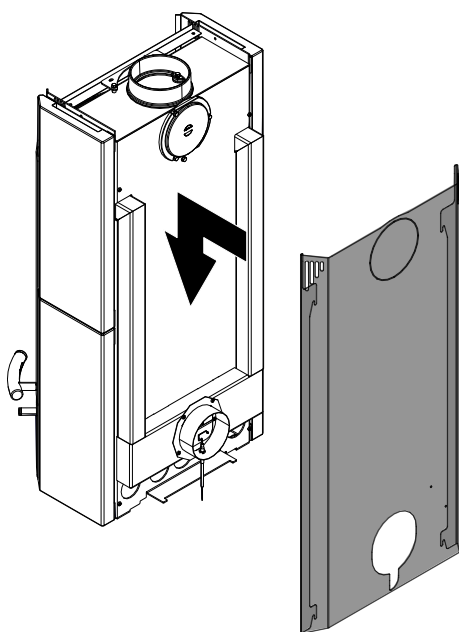
Abb. 34: Rückwand montieren
