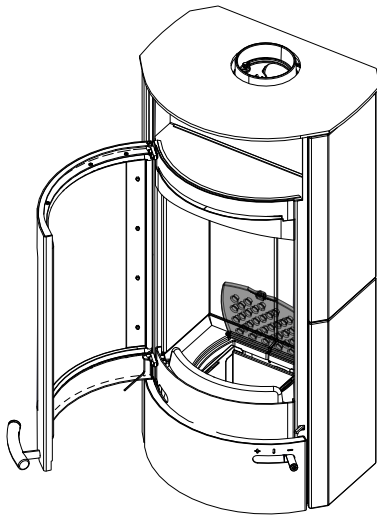
Abb. 46: Rost hochklappen
