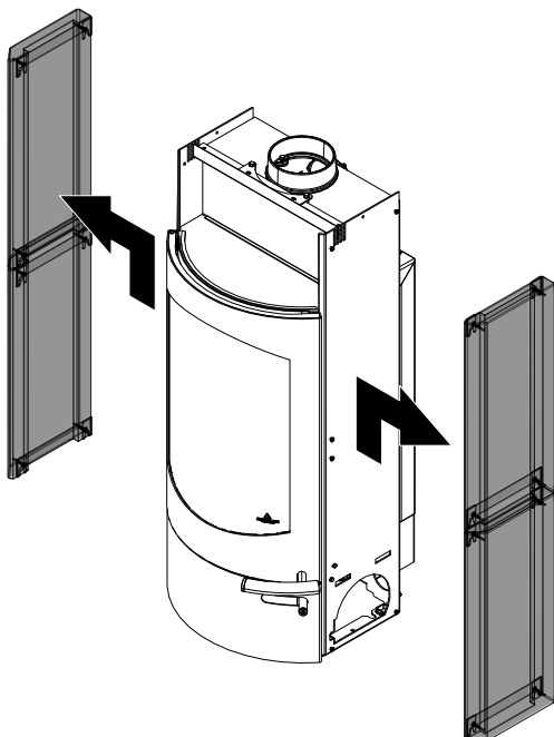
Abb. 51: Seitenverkleidung abnehmen
