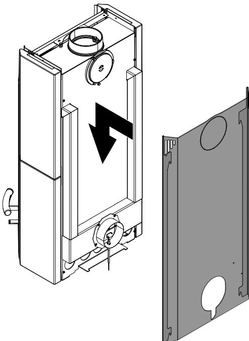
Abb. 14: Rückwand montieren
