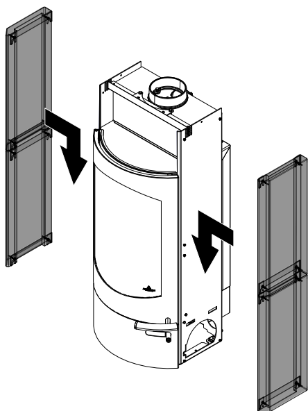
Abb. 33: Seitenverkleidung anbringen
