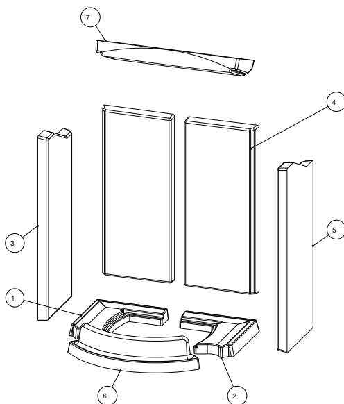
Abb. 16: Keramott einbauen
