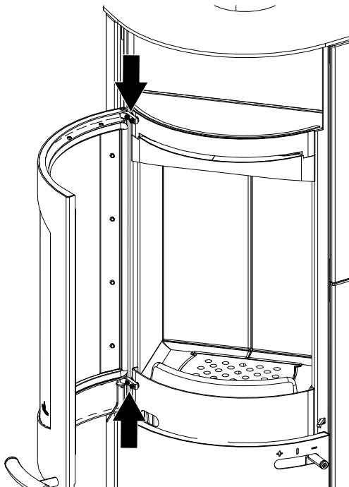
Abb. 37: Türeinstellschrauben
