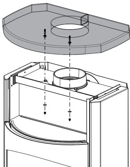
Abb. 28: Deckel montieren
