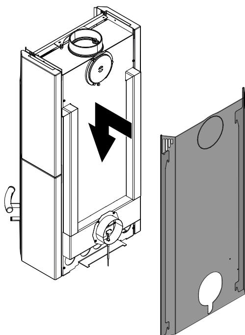
Abb. 55: Rückwand montieren
