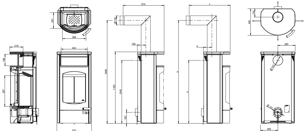
Abb. 2: Abmessungen
