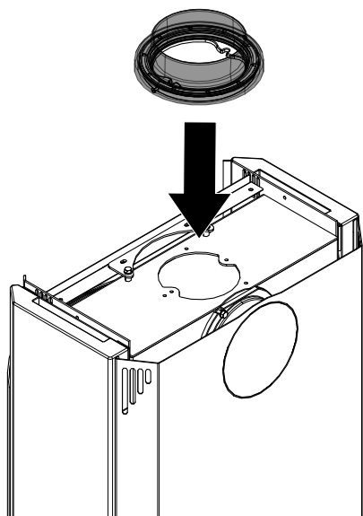
Abb. 21: Drehrauchrohrstutzen montieren
