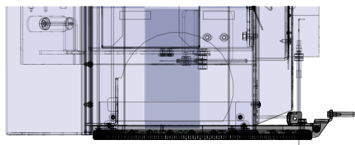
Abb. 24: Drehteller platzieren
