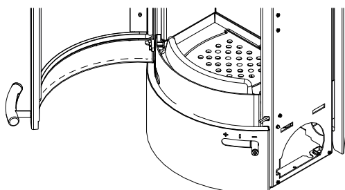
Abb. 40: Türverschluss einstellen
