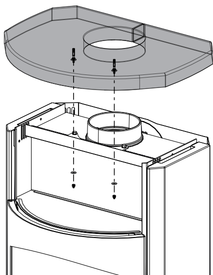
Abb. 35: Deckel montieren
