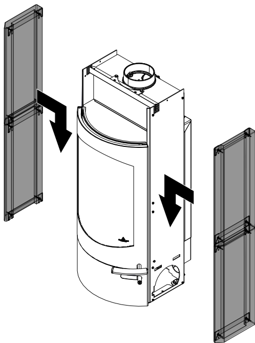
Abb. 54: Seitenverkleidung montieren
