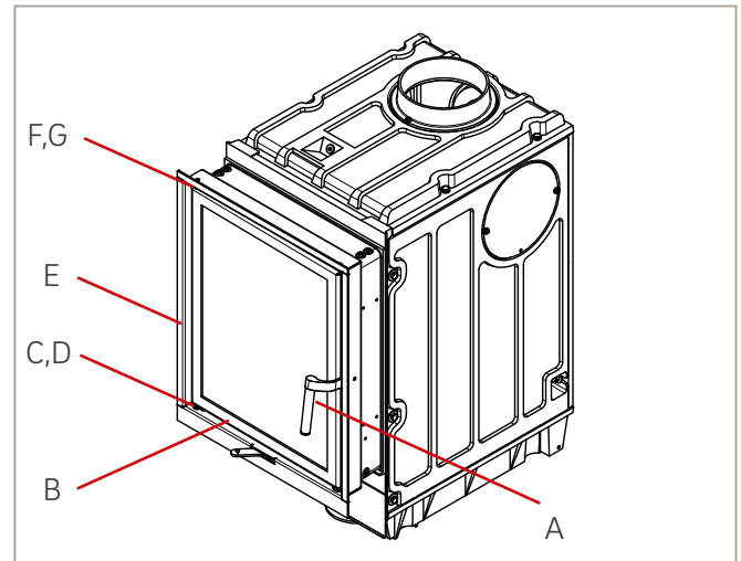
Abb. 4: Abbildung Demontage und Montage Fülltür - am Beispiel Profi K
