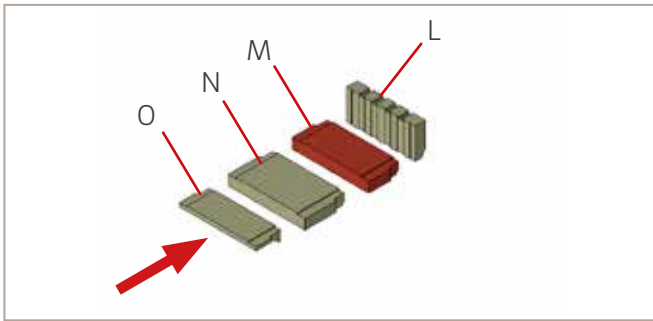
Abb. 53: Einbau Bauteile L, M, N, O
