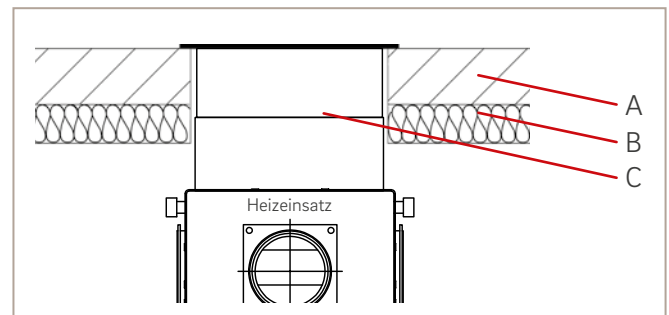
Abb. 66: Beispiel Wärmeschutzdämmung Außenbefeuerung
