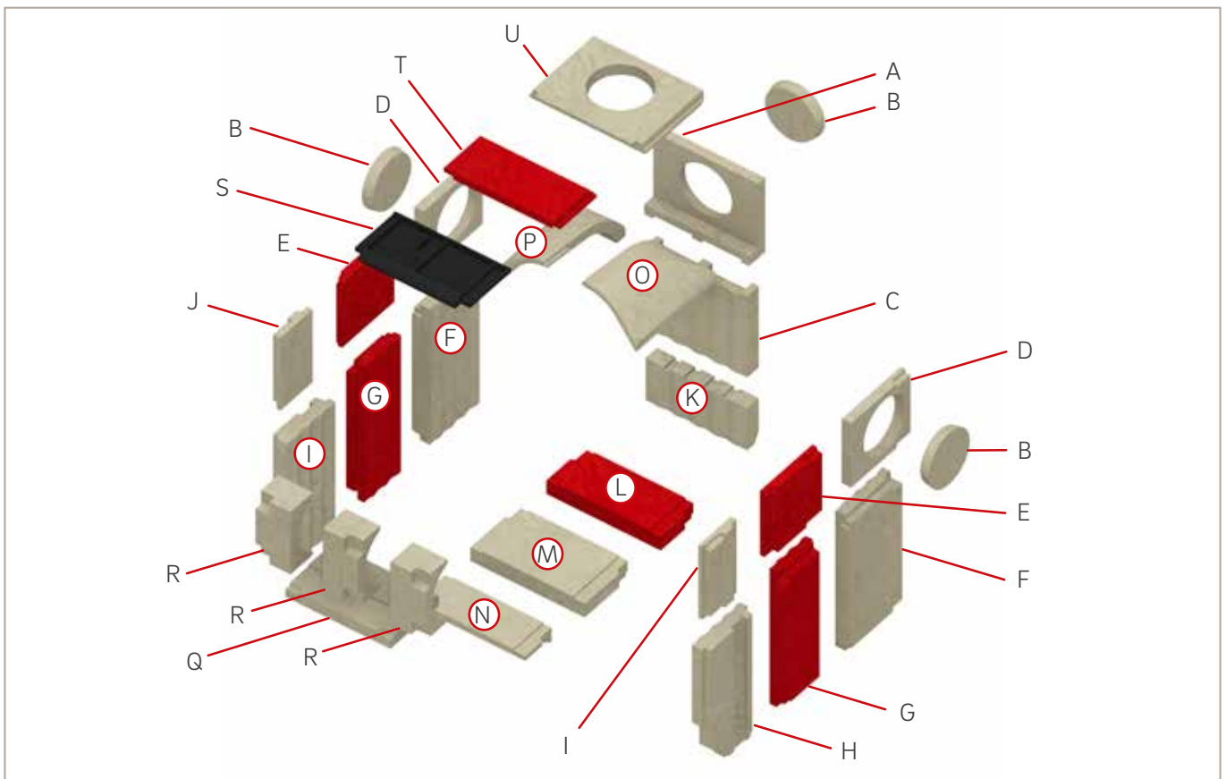
Abb. 45: Zusammenbau Innenauskleidung
