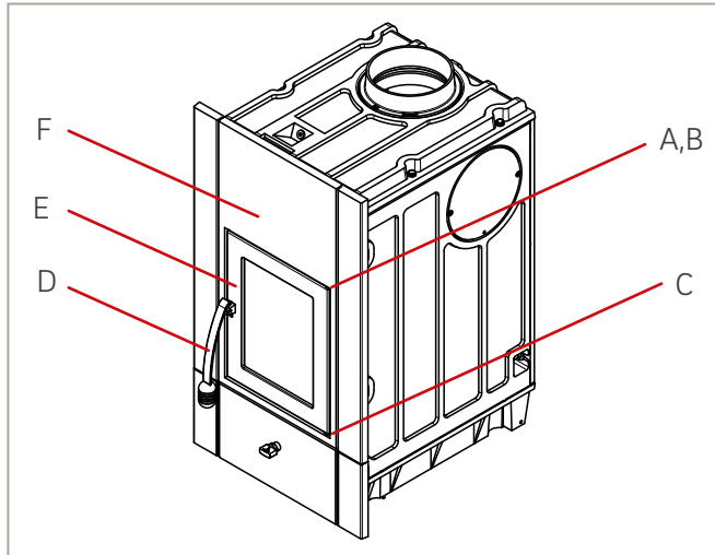
Abb. 17: Abbildung Demontage und Montage Fülltür
