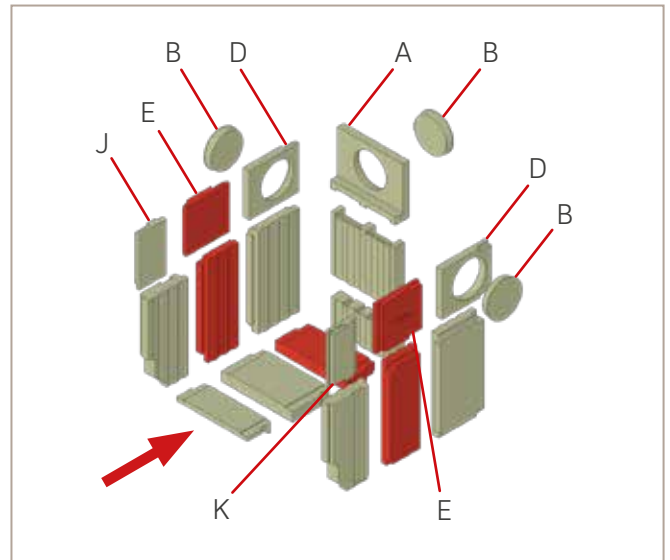
Abb. 55: Einbau Bauteile A, B, D, E, J, K
