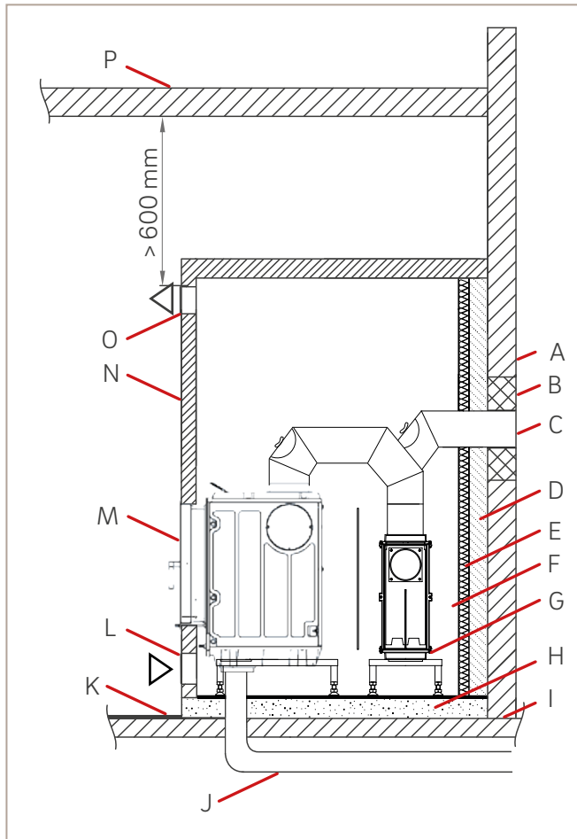
Abb. 62: Einbaubeispiel für einen Heizeinsatz vor zu schützenden Wänden, Böden, Decken
