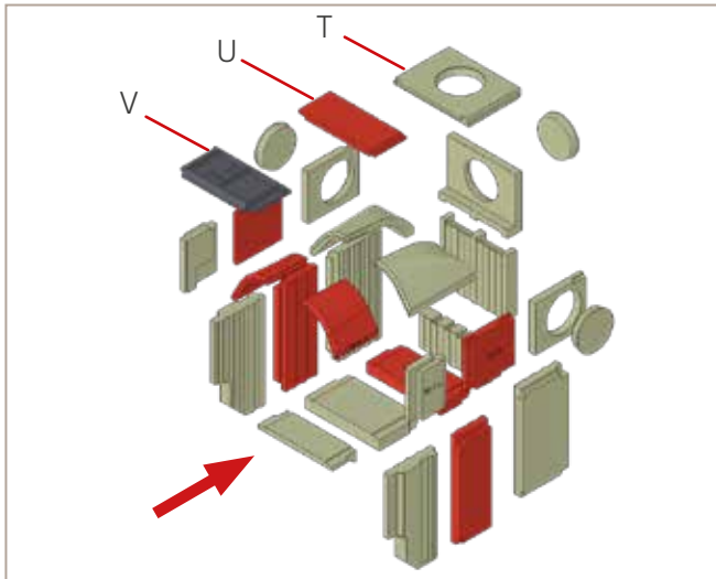
Abb.57: Einbau T, U, V
