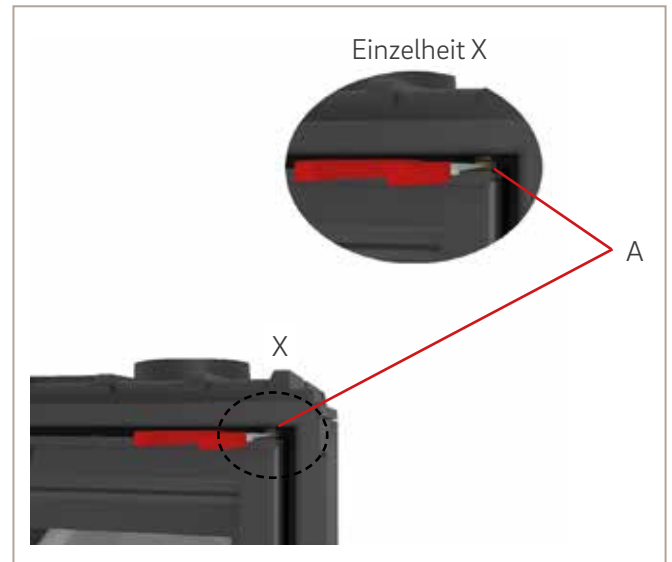
Abb. 16: Sicherungsclip setzen
