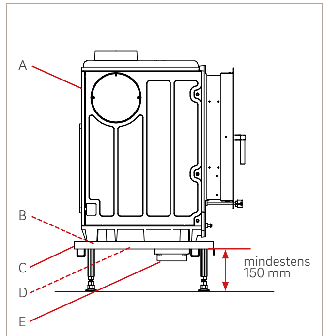
Abb. 25: Traglager, Profi K - minimaler Abstand
