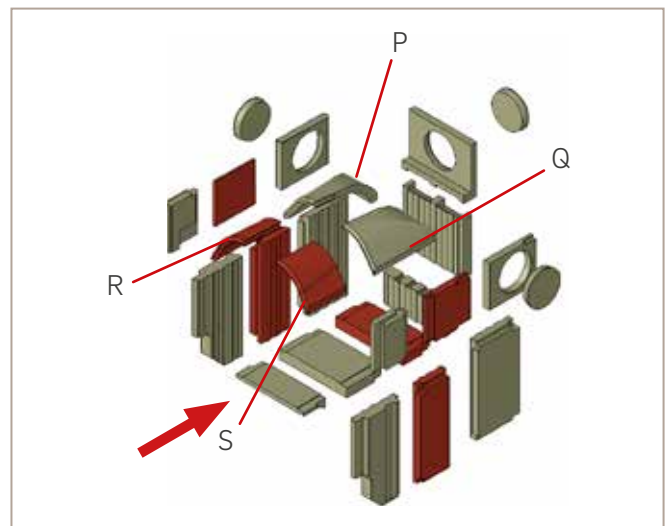
Abb. 56: Einbau Bauteile P, Q, R, S
