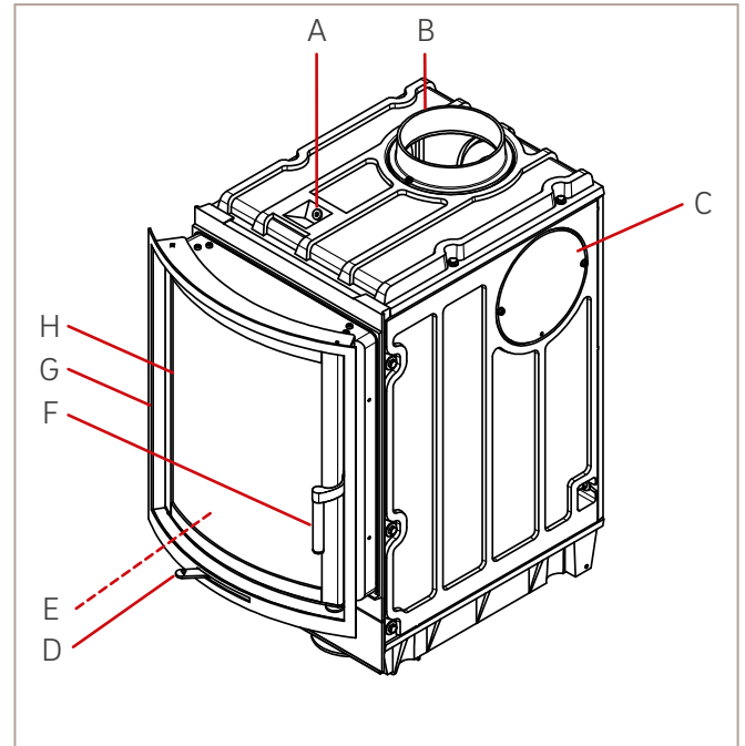
Abb. 3: Am Beispiel Profi K 7
