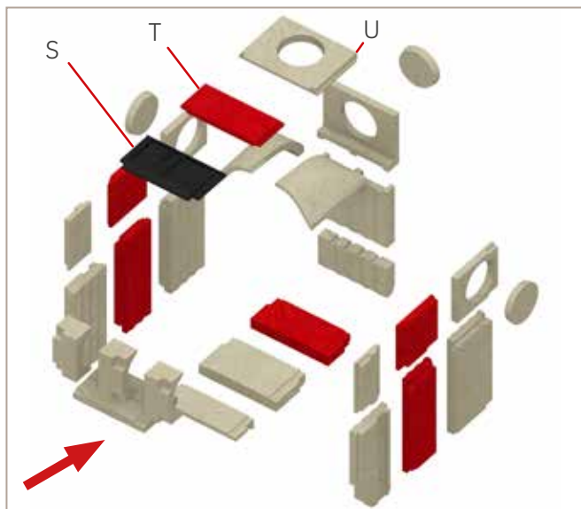
Abb.51: Einbau U, T, S
