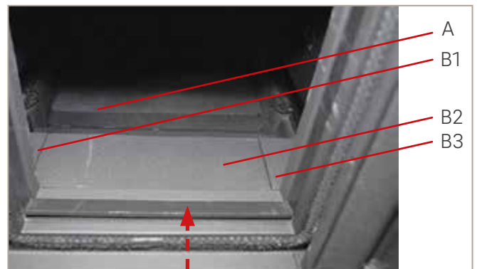
Abb. 41: Montage Primärluftkanäle
