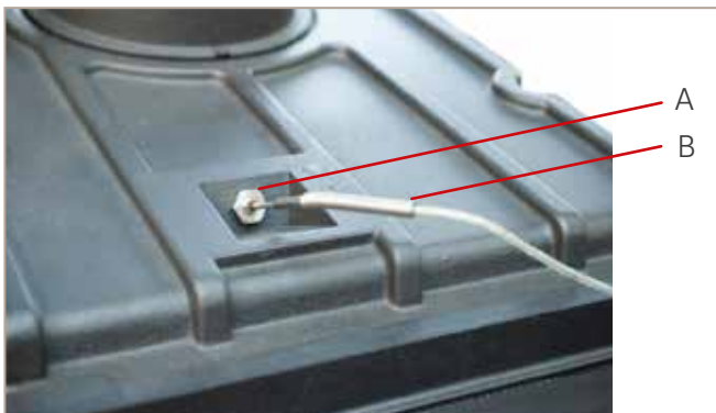
Abb. 60: SMR-Feuerraumfühler in Heizeinsatz montiert
