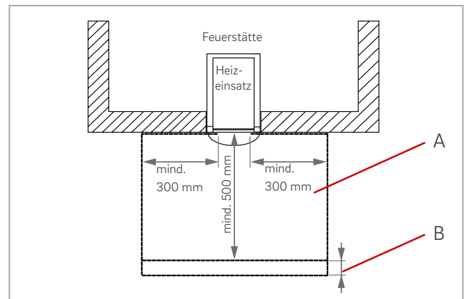
Abb. 63: Belag aus nicht brennbaren Baustoffen im Bereich vor der Feuerraumöffnung, Schema
