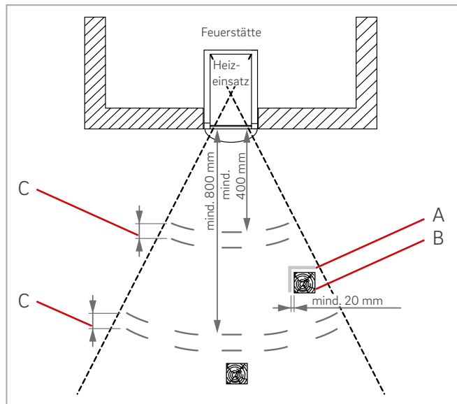
Abb. 64: Schutz von brennbaren Bauteilen im Strahlungsbereich vor der Feuerraumöffnung, Schema
