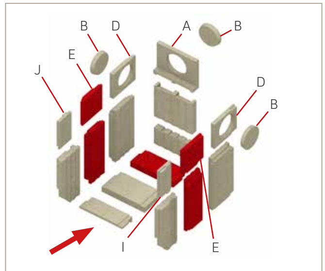
Abb. 48: Einbau Bauteile A, B, D, E, I, J
