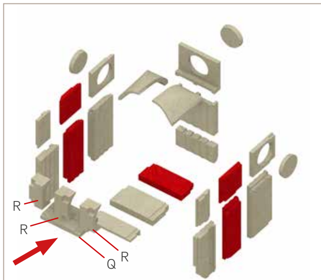
Abb.50: Einbau Q, R
