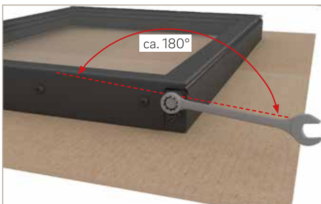
Abb. 11: Türfeder mit Maul-/Ringschlüssel vorspannen
