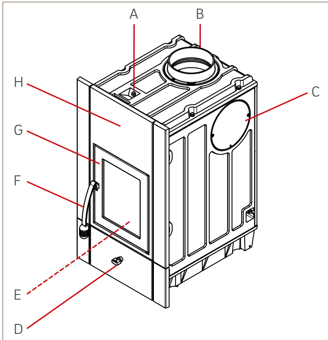
Abb. 2: Am Beispiel Profi 7 FP 480 x 830
