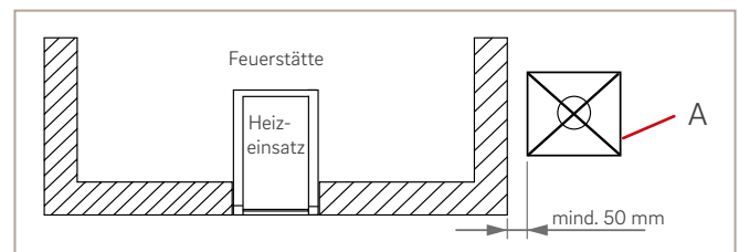
Abb. 65: Schutz und Abstände bei beheizten Flächen, Schema
