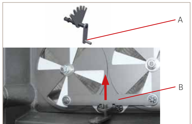
Abb. 33: Drehschieber und Welle, unten
