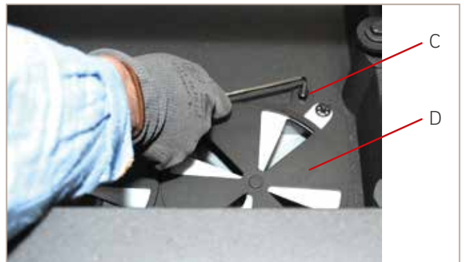
Abb. 32: Drehschieber ausbauen
