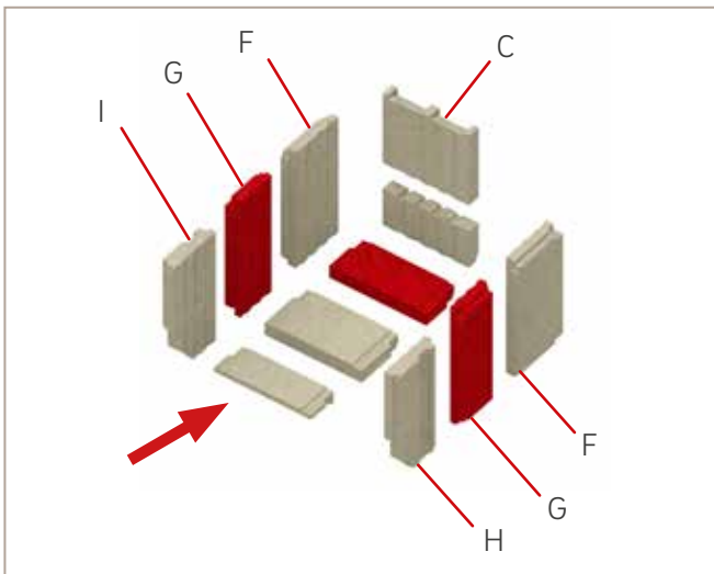
Abb. 47: Einbau Bauteile C, F, G, H, I
