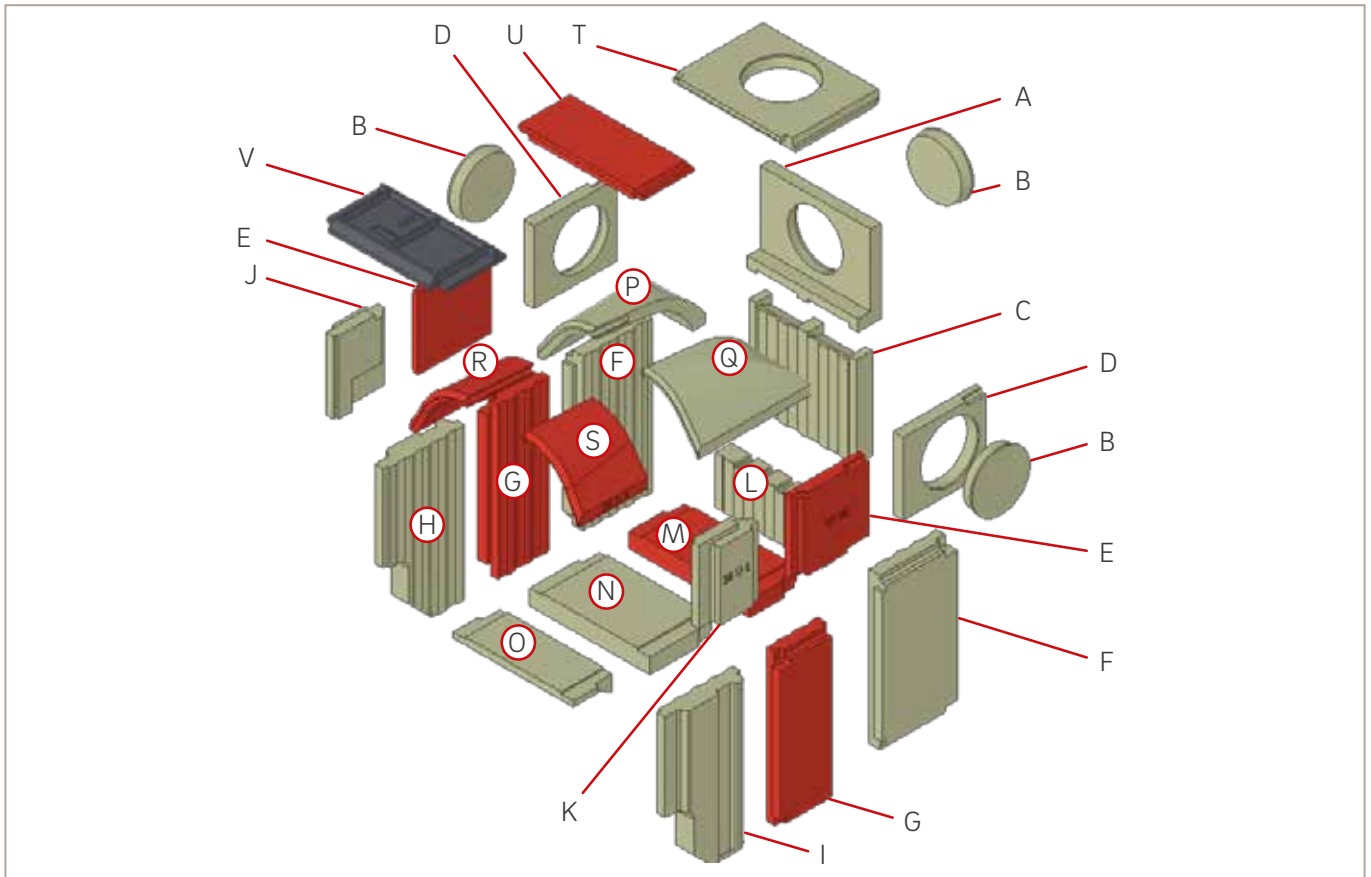
Abb. 52: Zusammenbau Innenauskleidung
