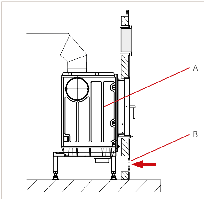
Abb. 28: Beispiel: Verbrennungsluftzufuhr aus dem Aufstellraum
