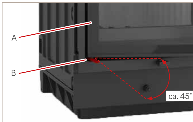
Abb. 7: Spannschlüssel ansetzen
