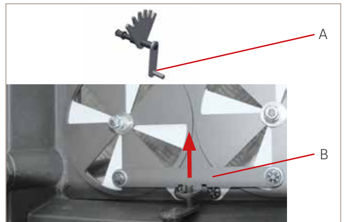
Abb. 61: Drehschieber und Welle, unten
