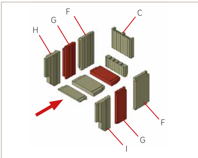
Abb. 54: Einbau Bauteile C, F, G, H, I
