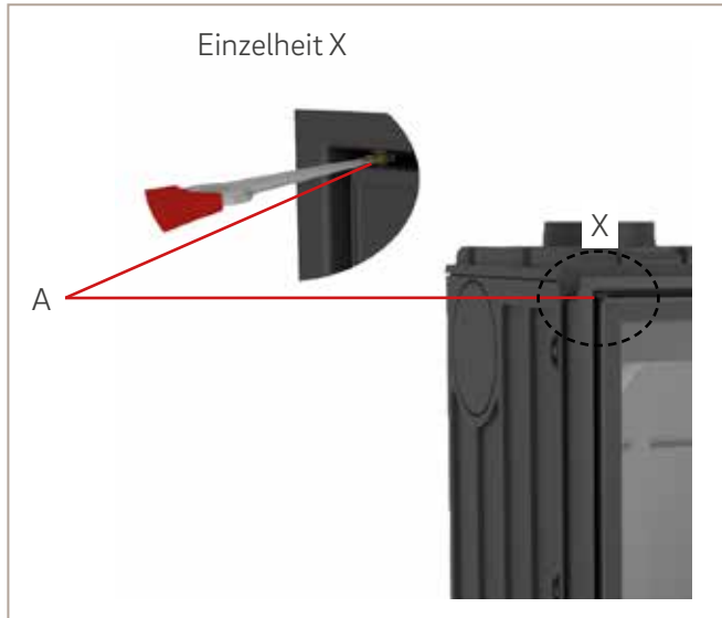
Abb. 6: Sicherungsclip abziehen
