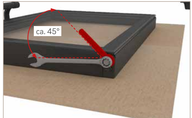
Abb. 12: Türfeder mit Spannschlüssel vorspannen
