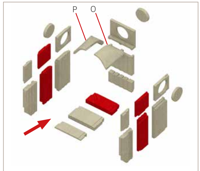
Abb. 49: Einbau Bauteile O, P
