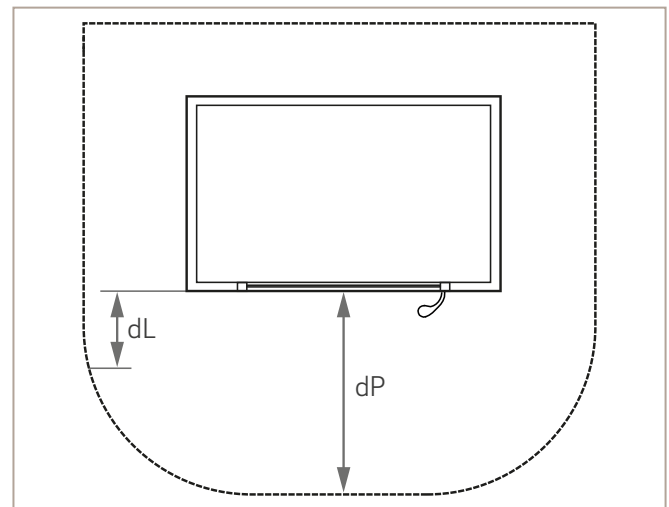
Abb. 5: Radius Strahlungsbereich
