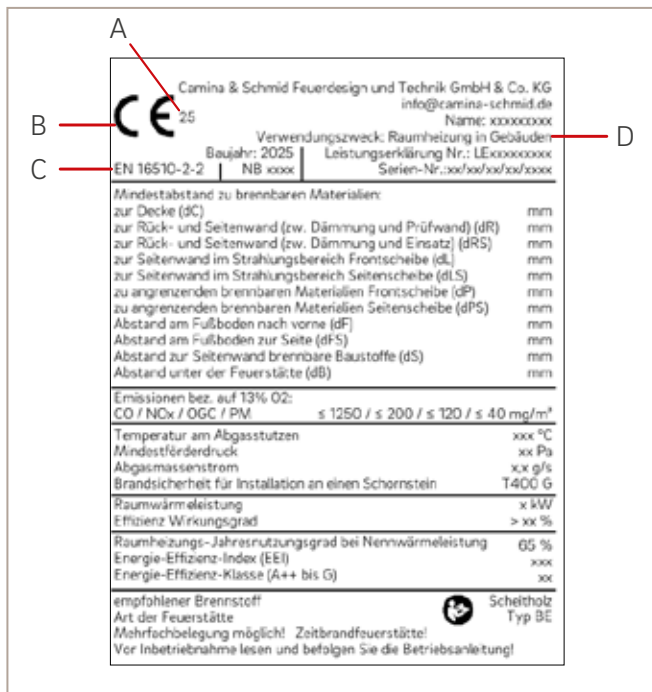
Abb. 1: Typenschild
