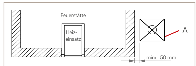
Abb. 6: Schutz und Abstände bei beheizten Flächen, Schema
