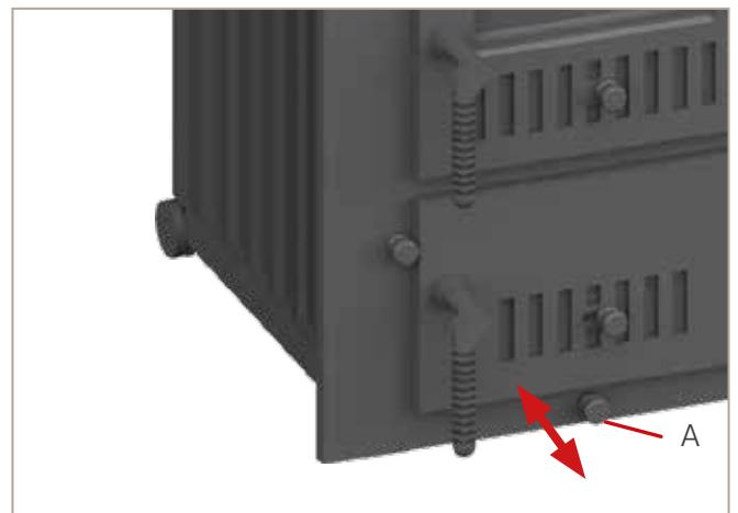
Abb. 19: Verbrennungsluftschieber 3
