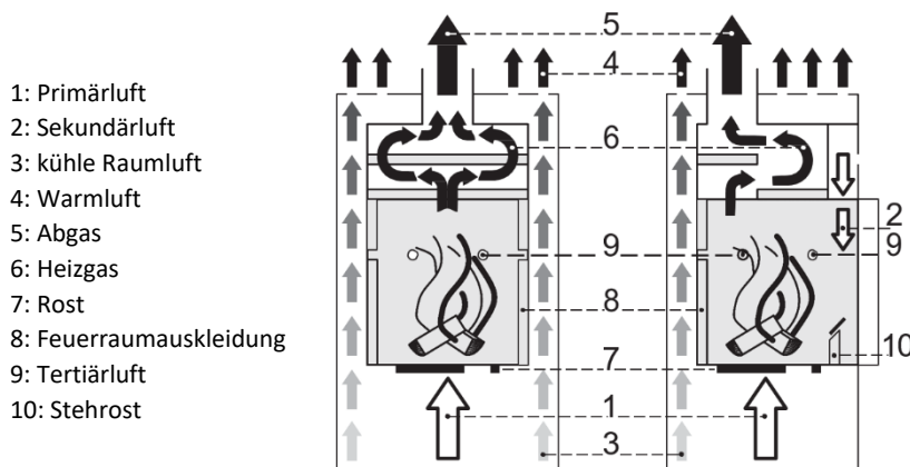
Abbildung 14 – Fire-Plus System, schematische Darstellung
