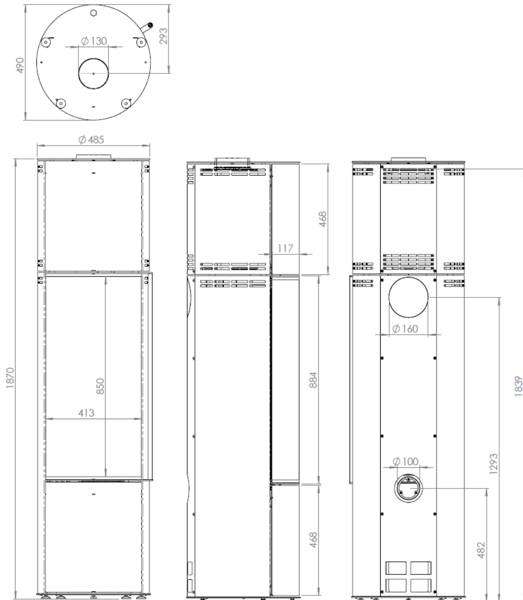
Abbildung 11 – Hauptmaße
