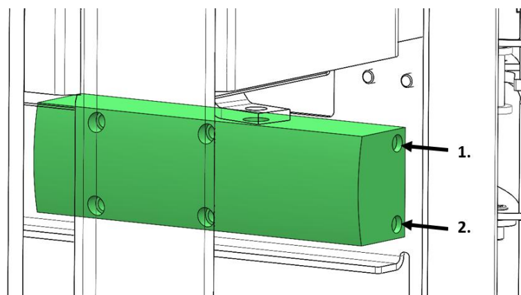
Abbildung 26 - Einstellung der Verschlussgeschwindigkeit
