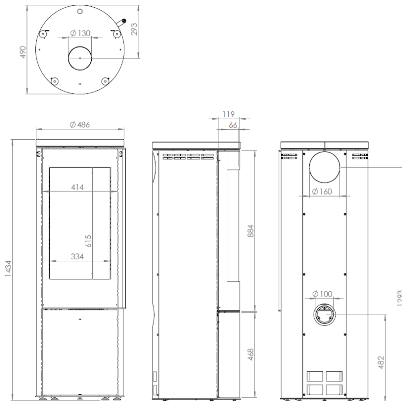
Abbildung 3 – Hauptmaße
