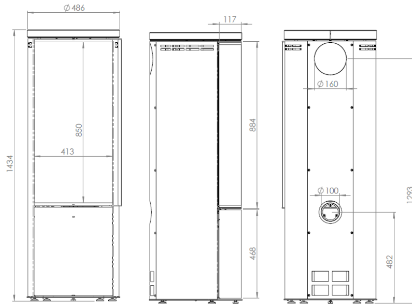
Abbildung 6 – Hauptmaße
