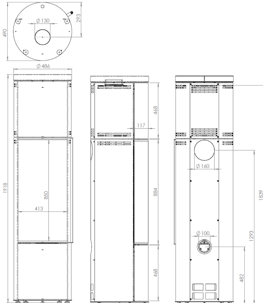
Abbildung 13 – Hauptmaße
