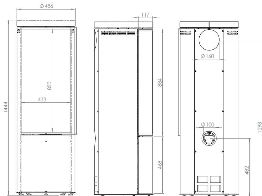
Abbildung 7 – Hauptmaße
