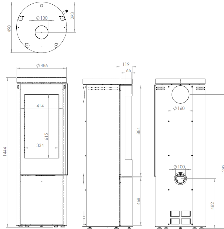
Abbildung 4 – Hauptmaße
