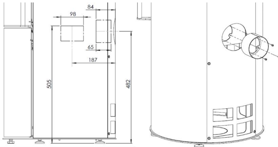
Abbildung 16- Verbrennungsluftanschluss
