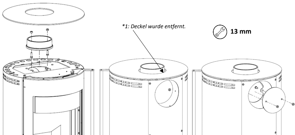
Abbildung 15 - Abgasstutzen und Abdeckung demontieren
