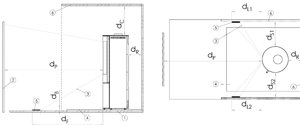
Abbildung 18 - Schematische Darstellung der Mindestabstände (siehe Tabelle 2)
