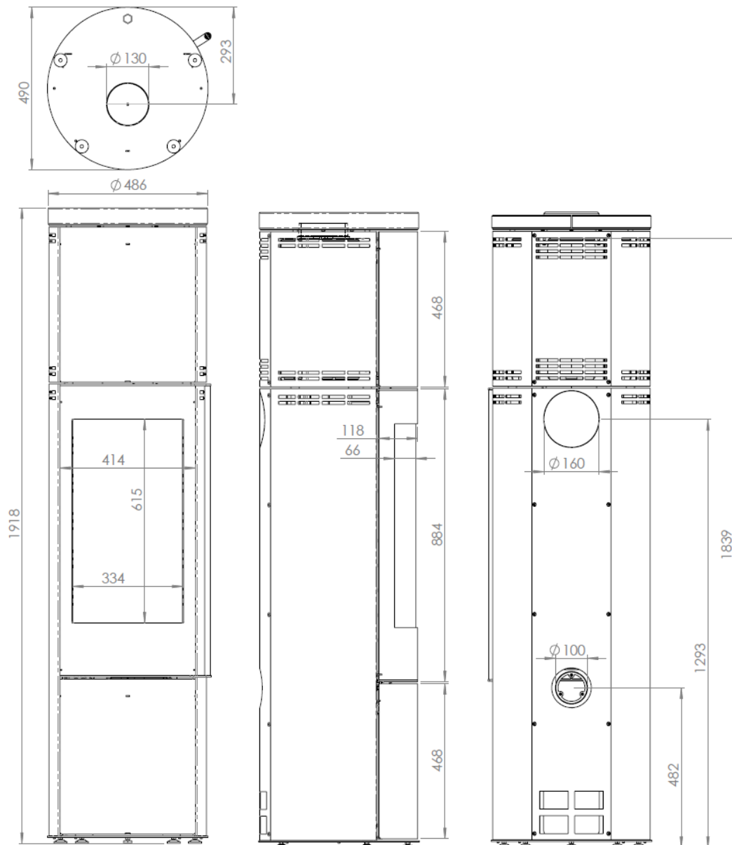
Abbildung 10 – Hauptmaße
