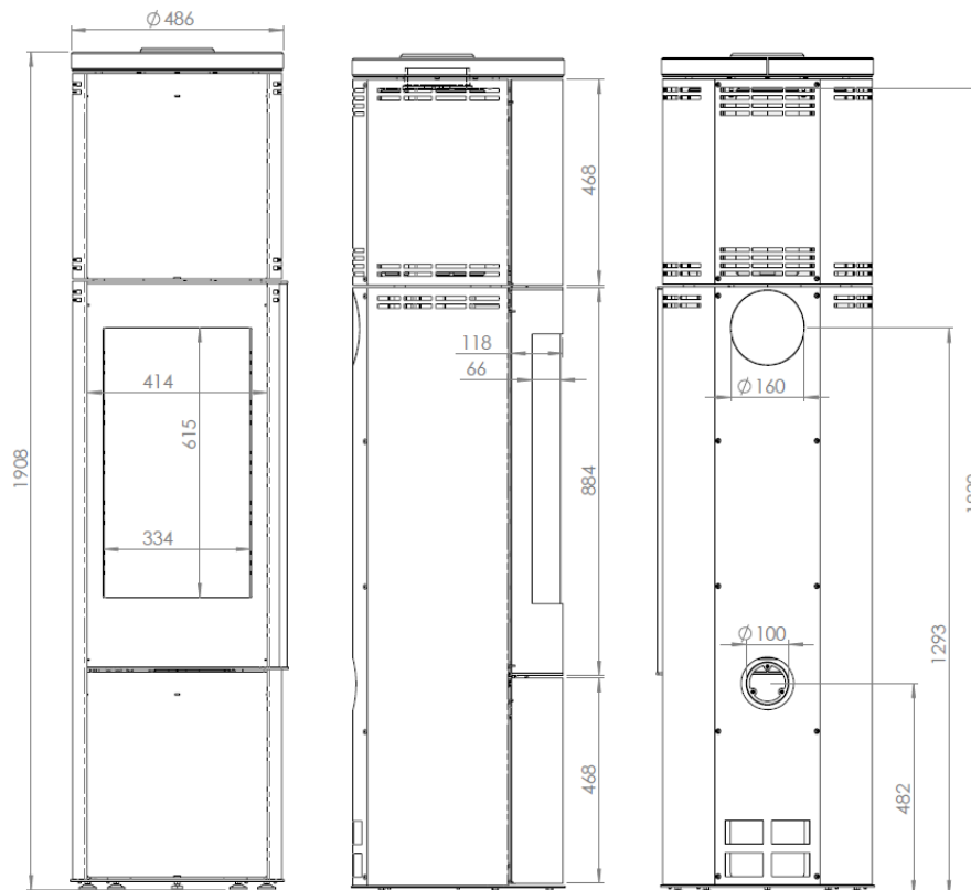
Abbildung 9 – Hauptmaße
