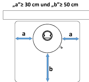
Abbildung 17 - Bodenplatte
