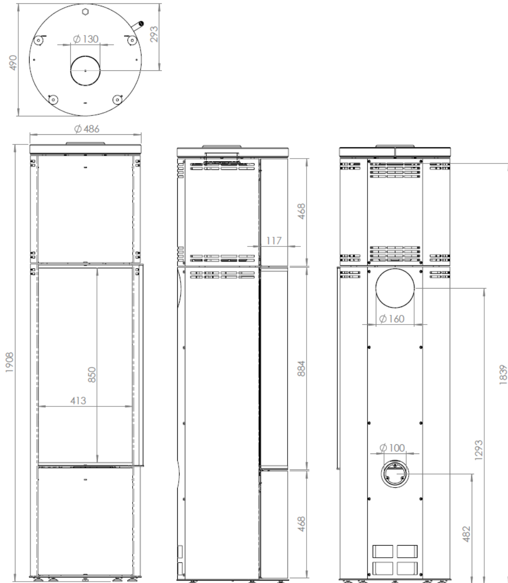
Abbildung 12 – Hauptmaße
