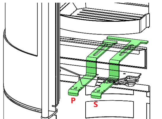
Abbildung 21 - P: Primärluftregler, S: Sekundärluftregler
