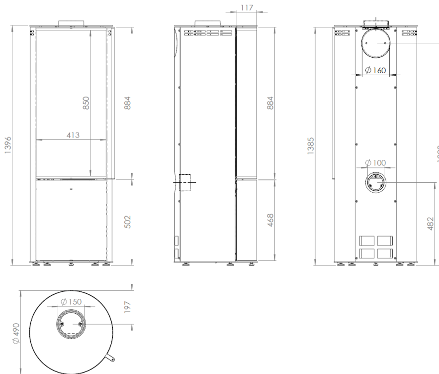
Abbildung 5 – Hauptmaße
