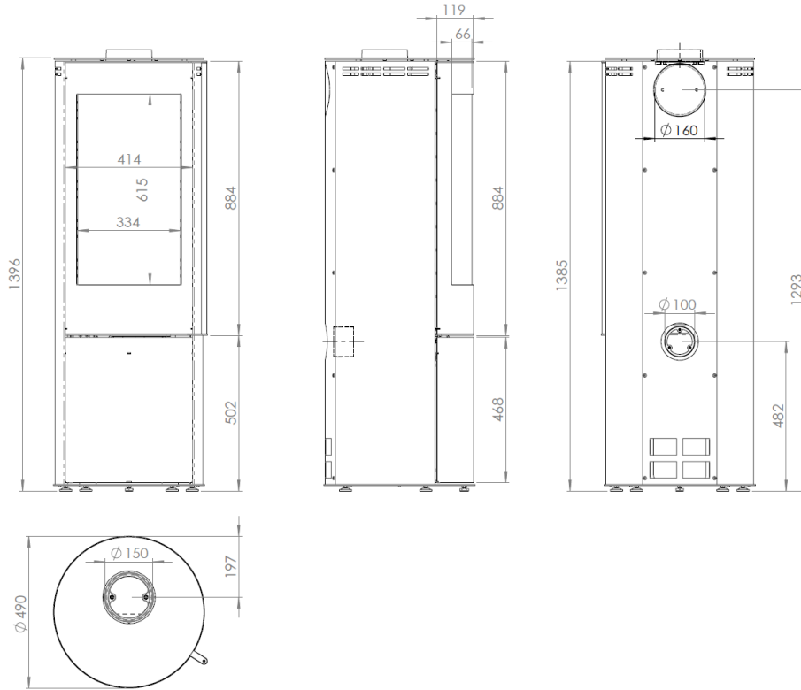
Abbildung 2 – Hauptmaße
