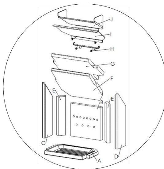
Abbildung 22 – Feuerraumauskleidung mit Rost
