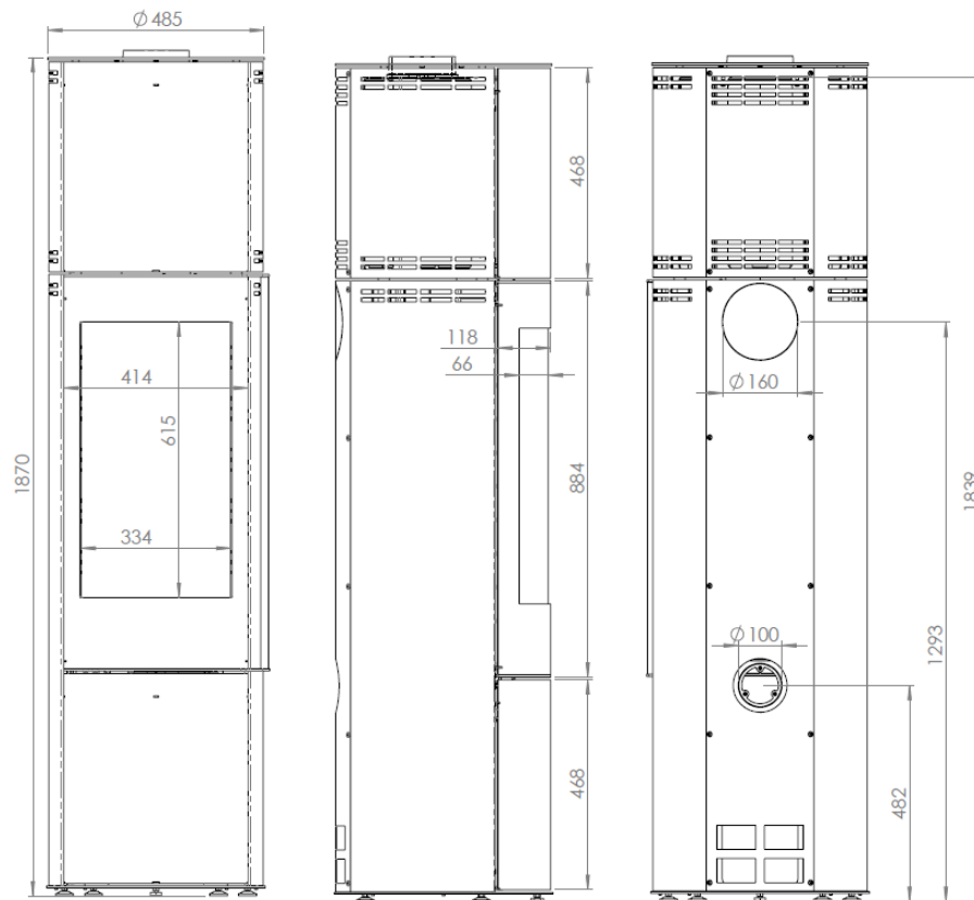
Abbildung 8 – Hauptmaße
