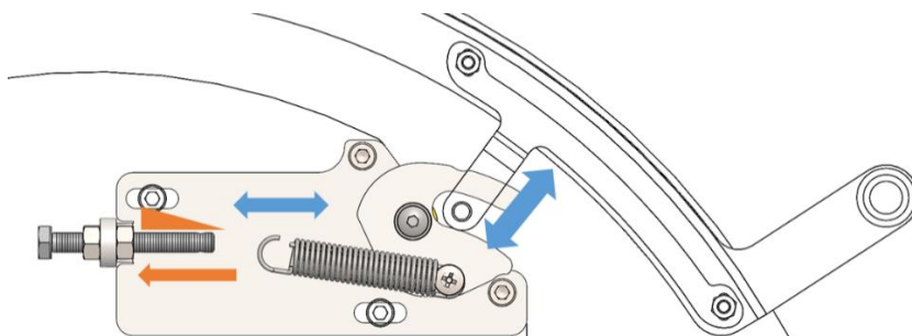
Abbildung 24 – Schnappverschluss
