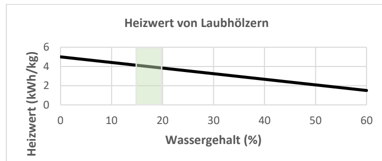
Abbildung 19 - Heizwertänderung in Abhängigkeit vom Wassergehalt
