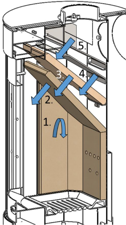
Abbildung 23 – Zugang zum Rauchraum
