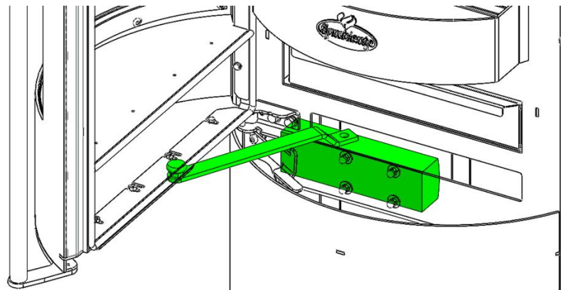
Abbildung 25 - Hydraulischer Türverschluss
