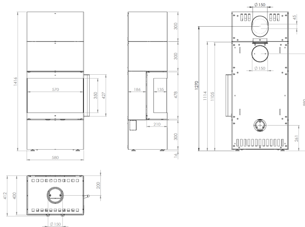
Abbildung 3 – Hauptmaße
