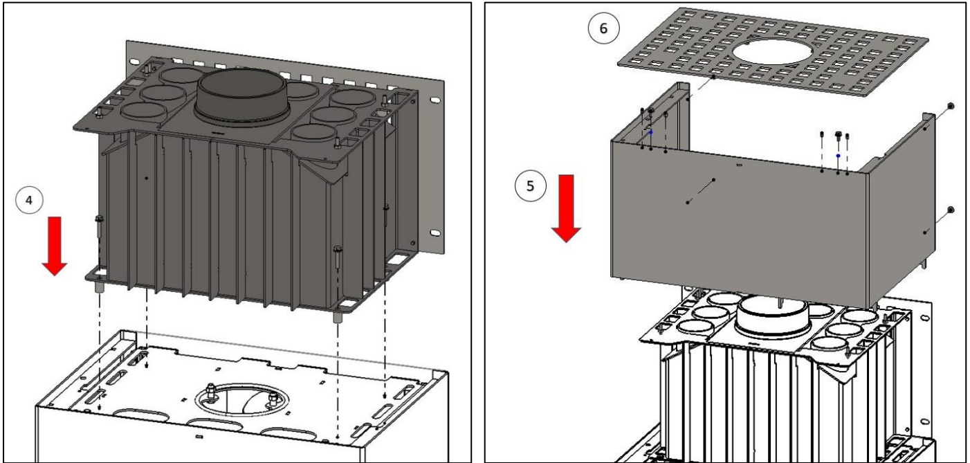
Abbildung 24 – Montage des Wärmetauschermoduls
