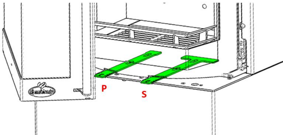
Abbildung 30 - P: Primärluftregler, S: Sekundärluftregler
