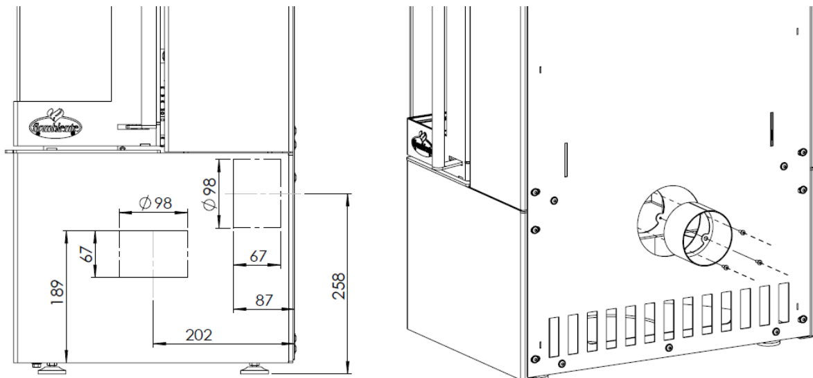
Abbildung 21 - Verbrennungsluftanschluss
