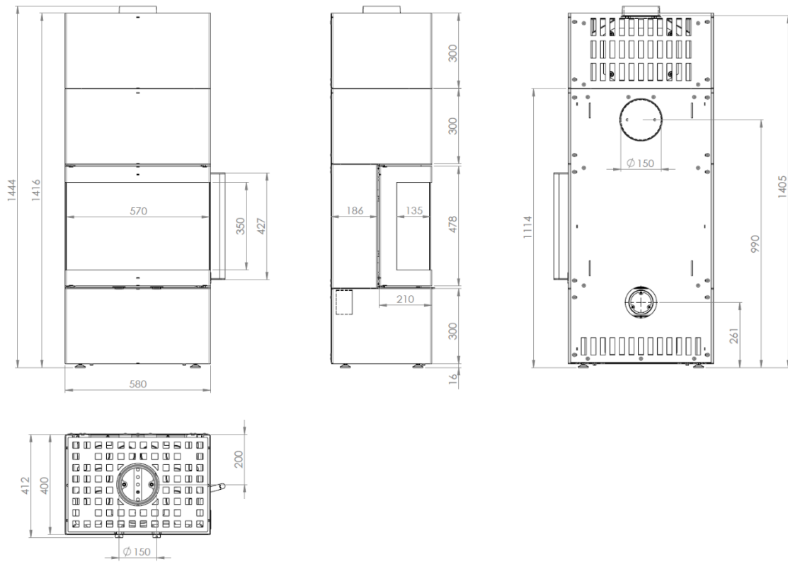
Abbildung 12 – Hauptmaße
