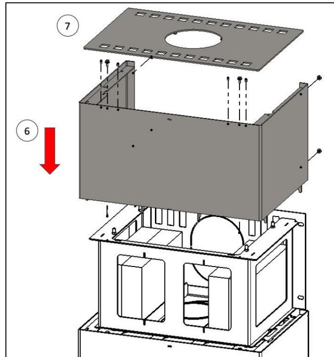
Abbildung 23-Montage des Wärmespeichermoduls
