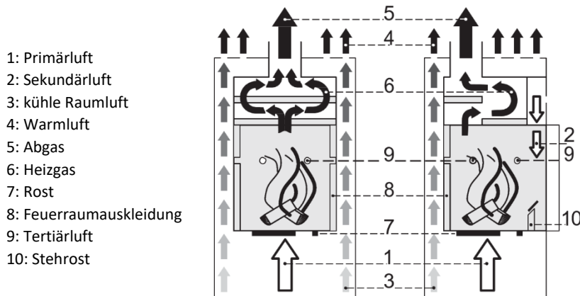
Abbildung 19 – Fire-Plus System, schematische Darstellung
