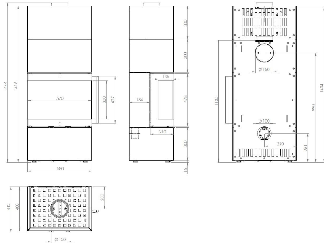
Abbildung 14 – Hauptmaße
