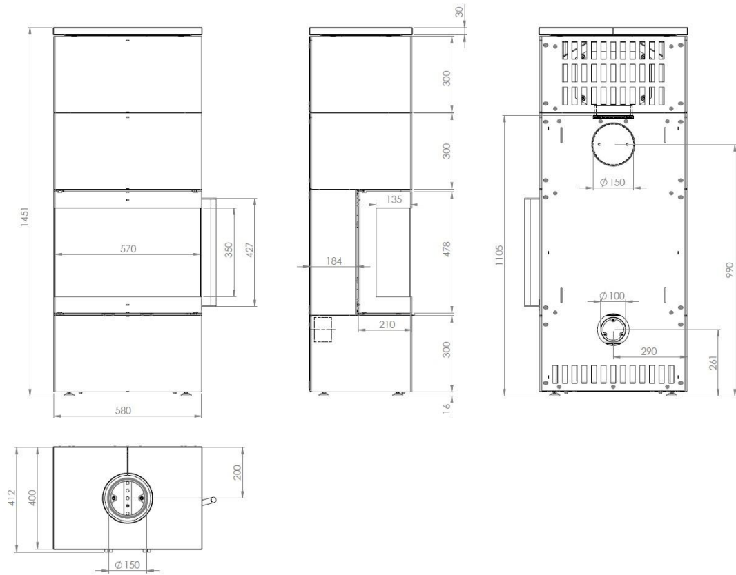
Abbildung 16 – Hauptmaße
