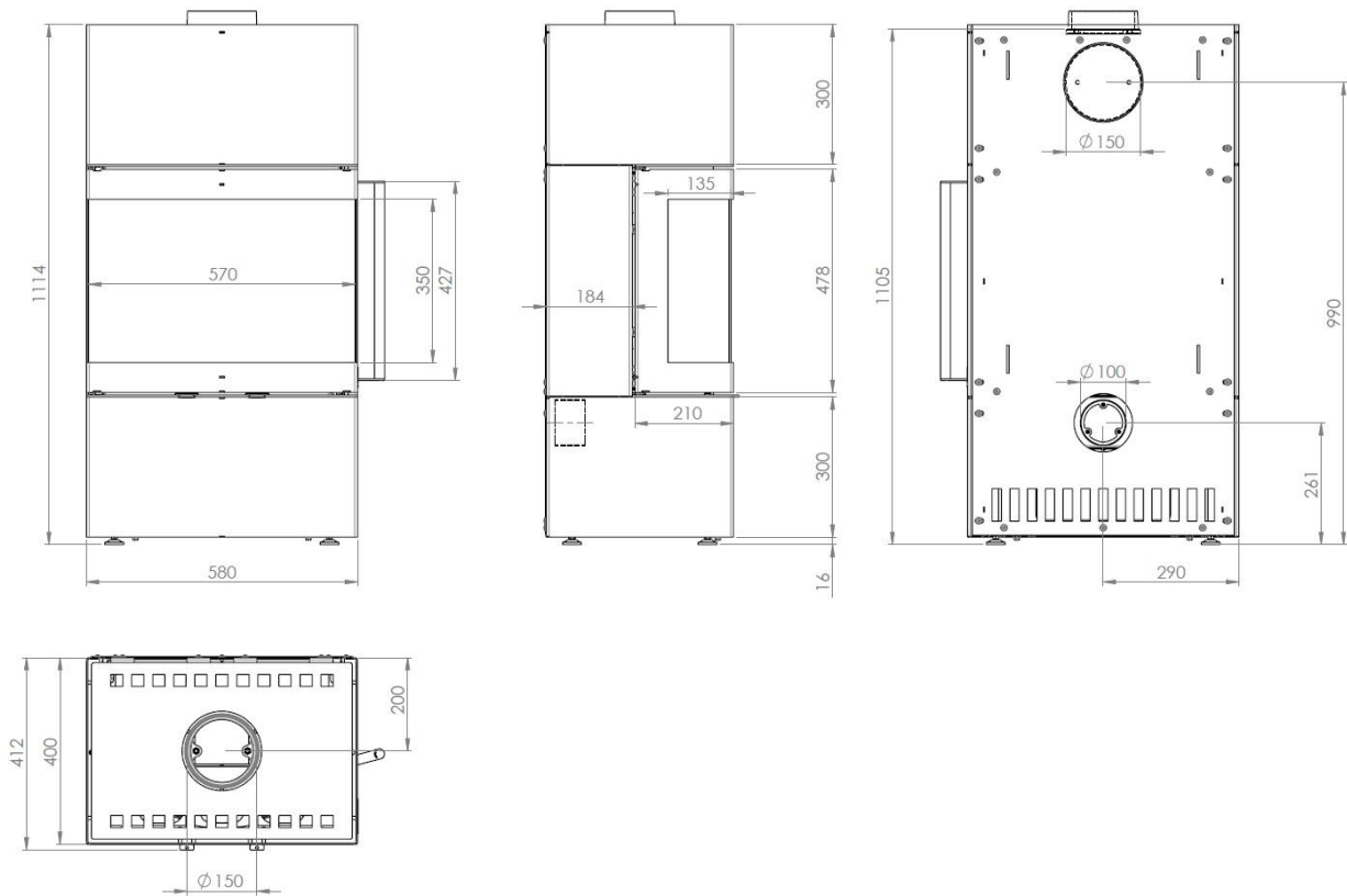
Abbildung 2 – Hauptmaße
