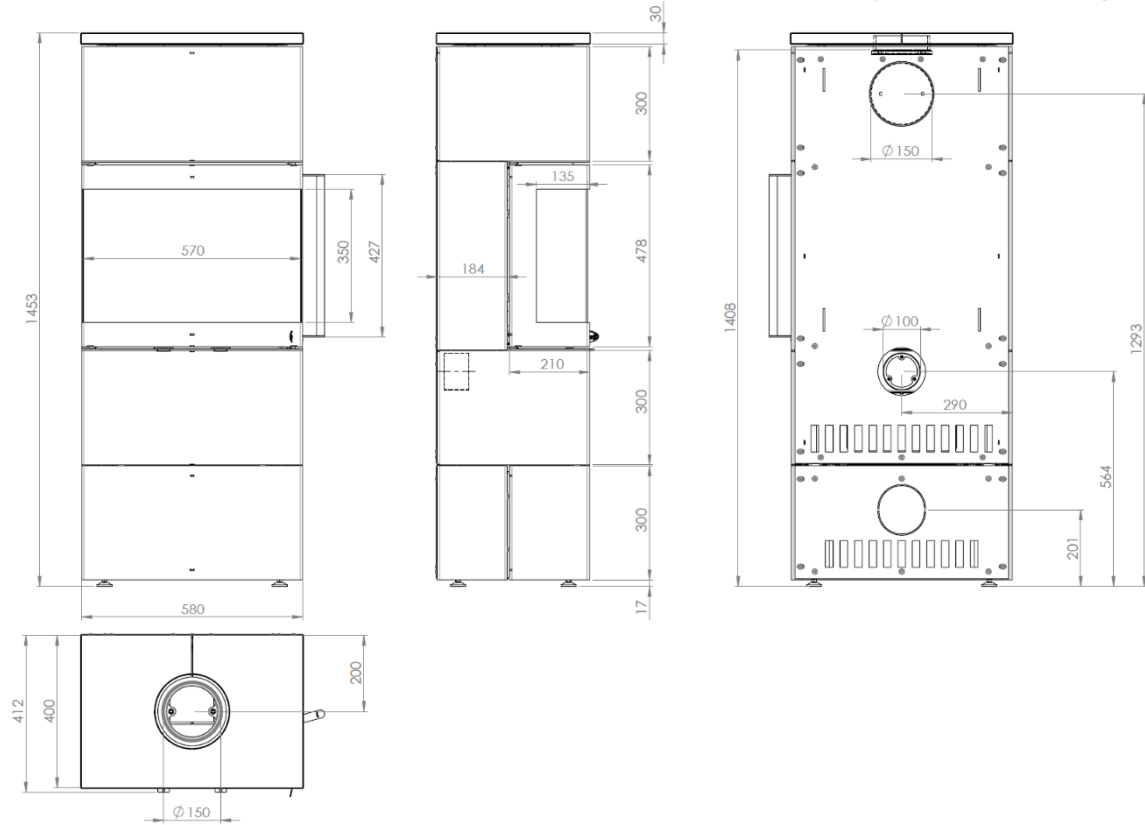
Abbildung 11 – Hauptmaße
