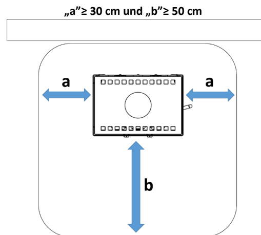
Abbildung 25 - Bodenplatte
