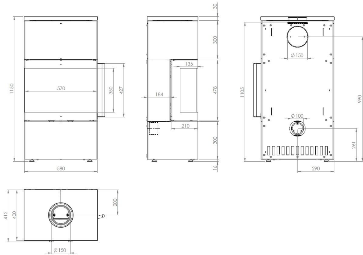
Abbildung 10 – Hauptmaße
