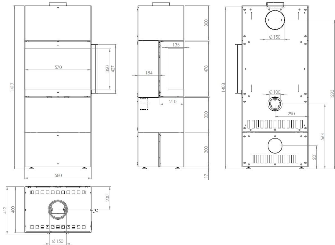
Abbildung 4 - Hauptmaße
