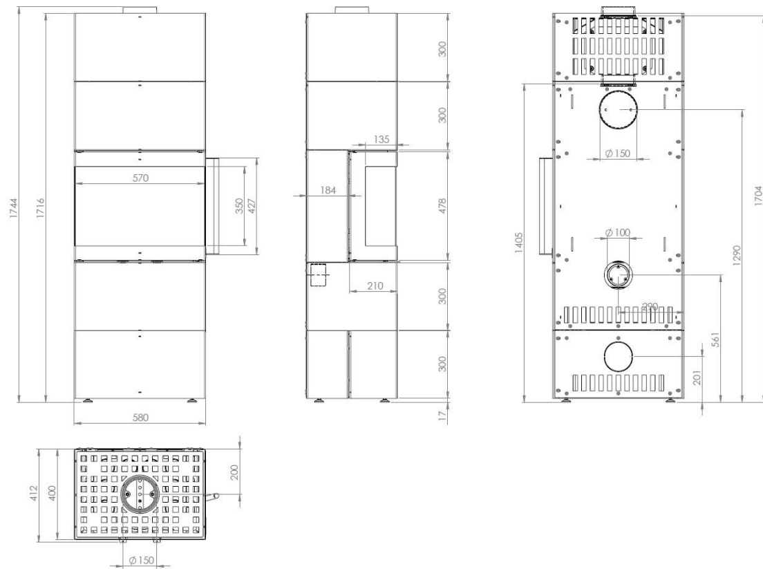
Abbildung 13 – Hauptmaße
