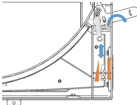
Abbildung 34 – Türschloss
