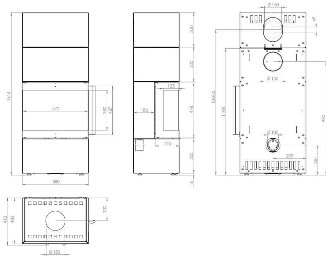
Abbildung 7 – Hauptmaße
