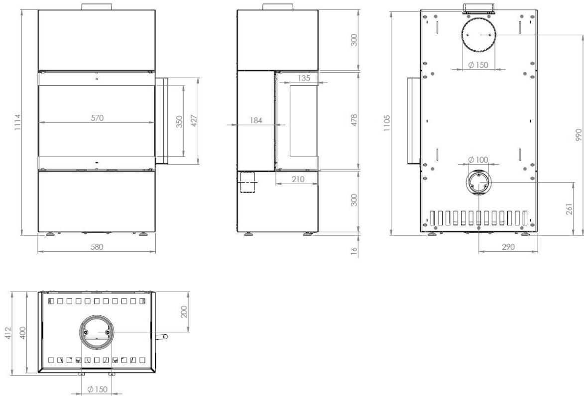
Abbildung 6 – Hauptmaße
