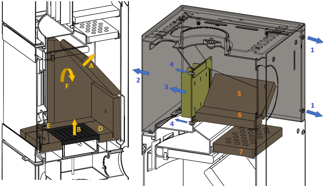
Abbildung 33 – Zugang zum Rauchraum
