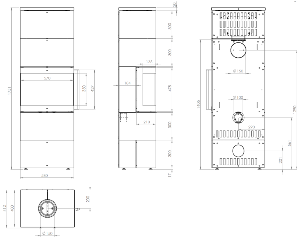
Abbildung 17 – Hauptmaße
