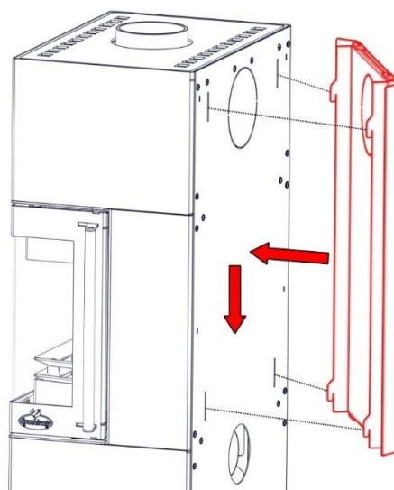
Abbildung 27 – Montage des Hitzeschutzblechs
