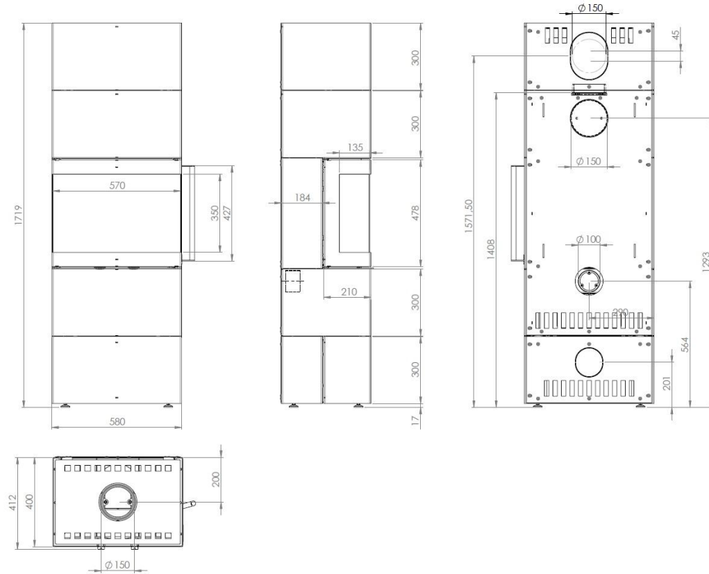
Abbildung 5 - Hauptmaße
