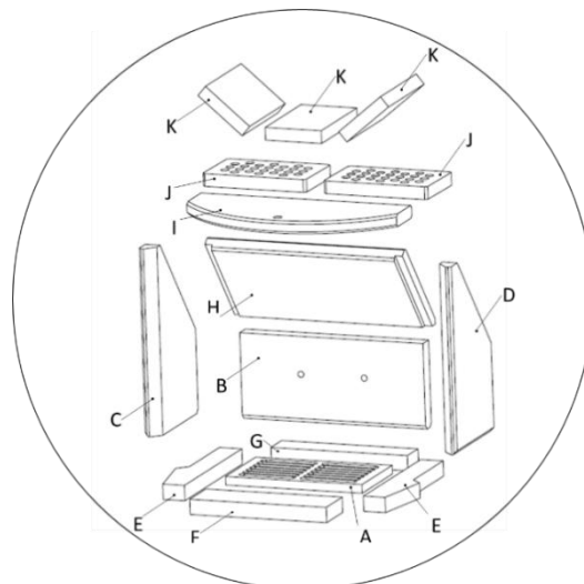
Abbildung 31 – Feuerraumauskleidung mit Rost
