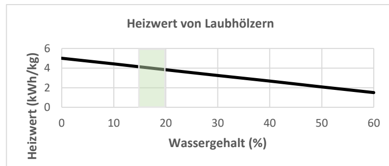
Abbildung 28 - Heizwertänderung in Abhängigkeit vom Wassergehalt
