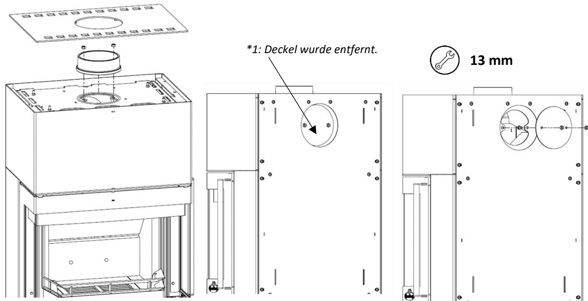
Abbildung 20 - Abgasstutzen und Abdeckung demontieren
