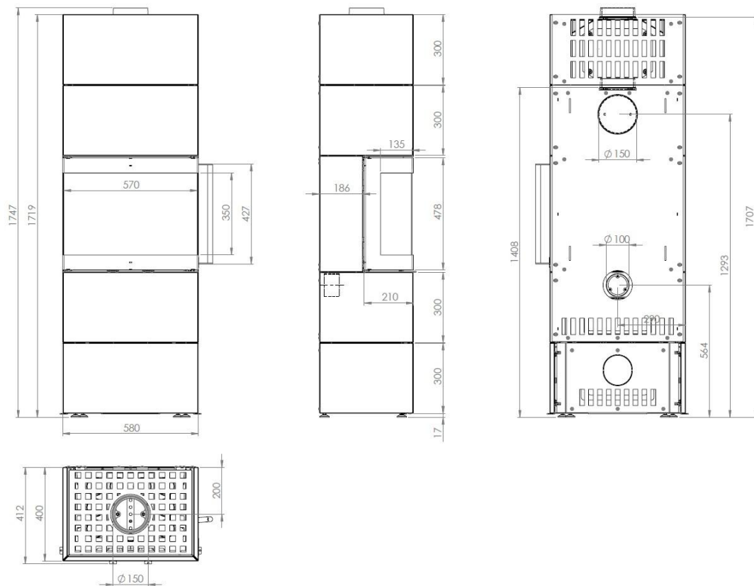
Abbildung 15 – Hauptmaße
