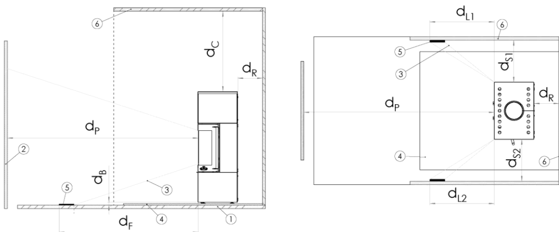
Abbildung 26 - Schematische Darstellung der Mindestabstände (siehe Tabelle 2)
