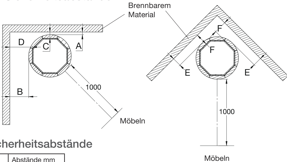
Sicherheitsabstände für die Aufstellung einer Nivellierbasis
