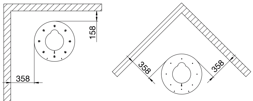
Sicherheitsabstände für die Aufstellung einer Nivellierbasis
