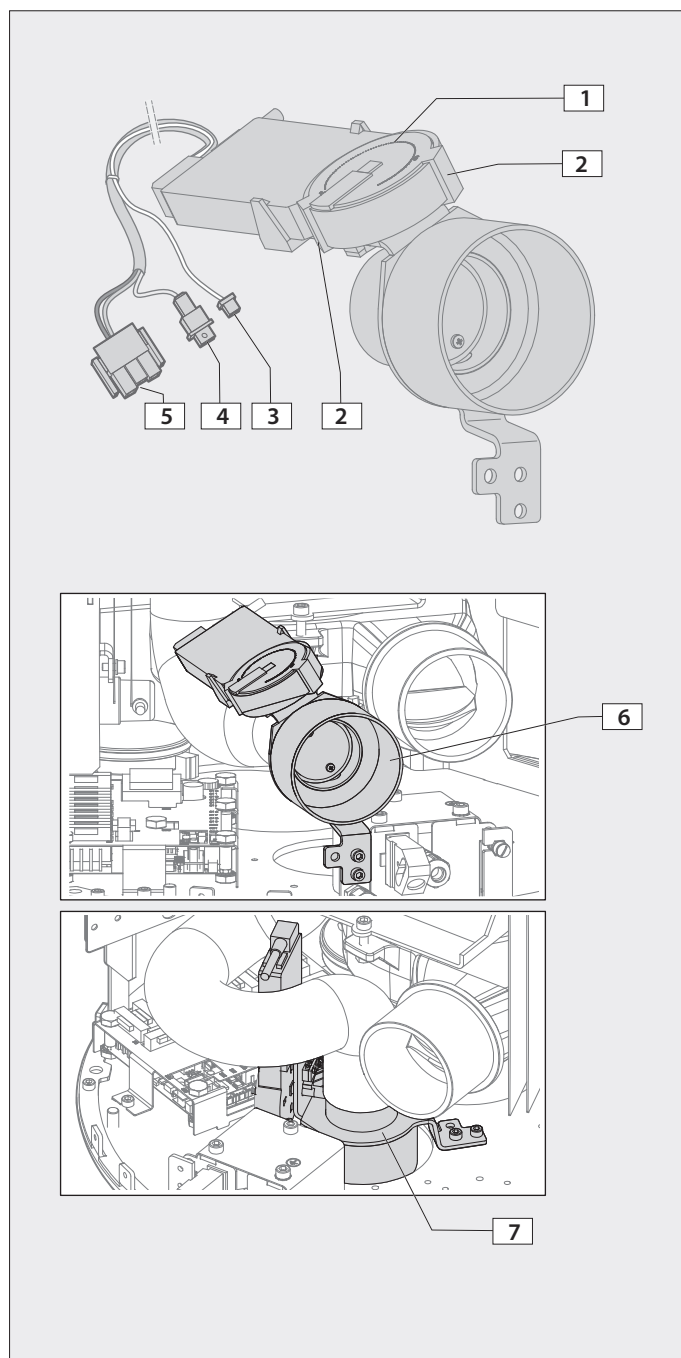
Abb. 2.13 Anschluss einer motorgesteuerten Verbrennungsluftklappe
