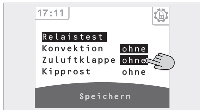
Abb. 2.20 Funktionsprüfung im Menü Relaistest
