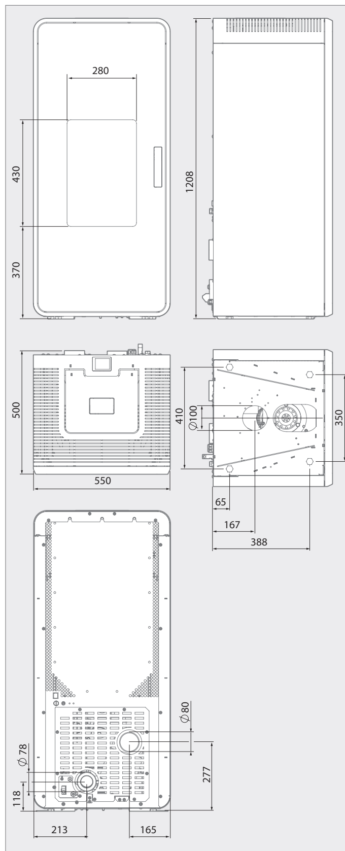
Abb. 2.4 Maße VESTA
