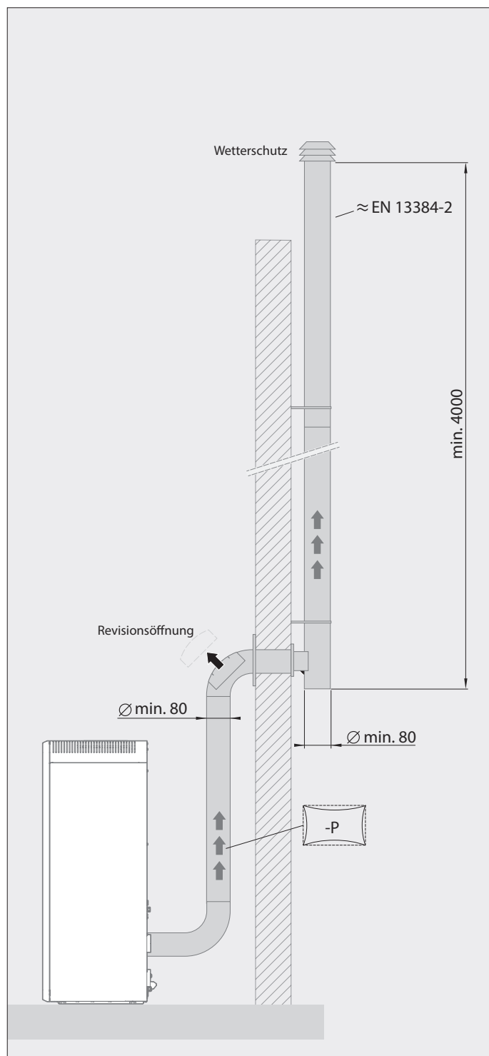
Fig. 2.6 Raccordement des gaz de combustion
