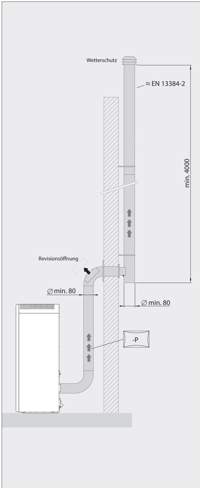
Abb. 2.6 Abgasanschluss
