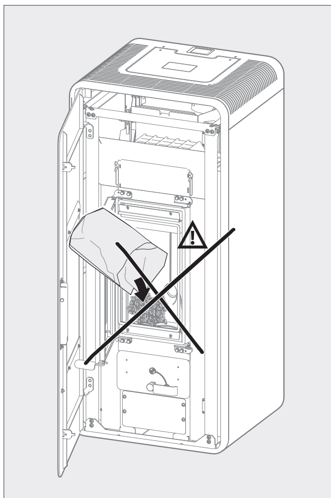
Abb. 3.7 Pellets nicht manuell in die Brennermulde füllen, außer nach leer gelaufenem Tank
