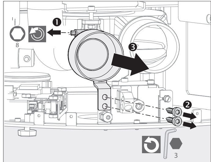
Abb. 2.15 Verbrennungsluftstutzen abschrauben
