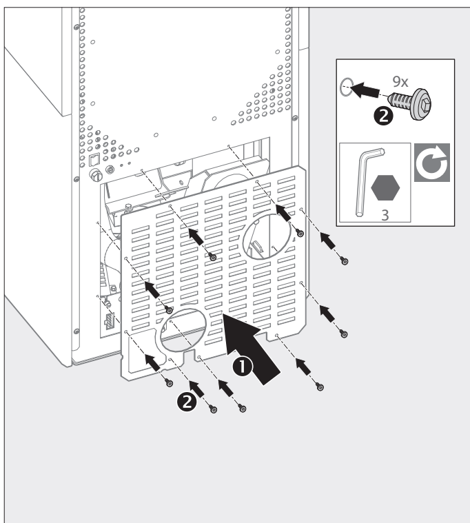
Fig. 2.12 Monter la paroi arrière
