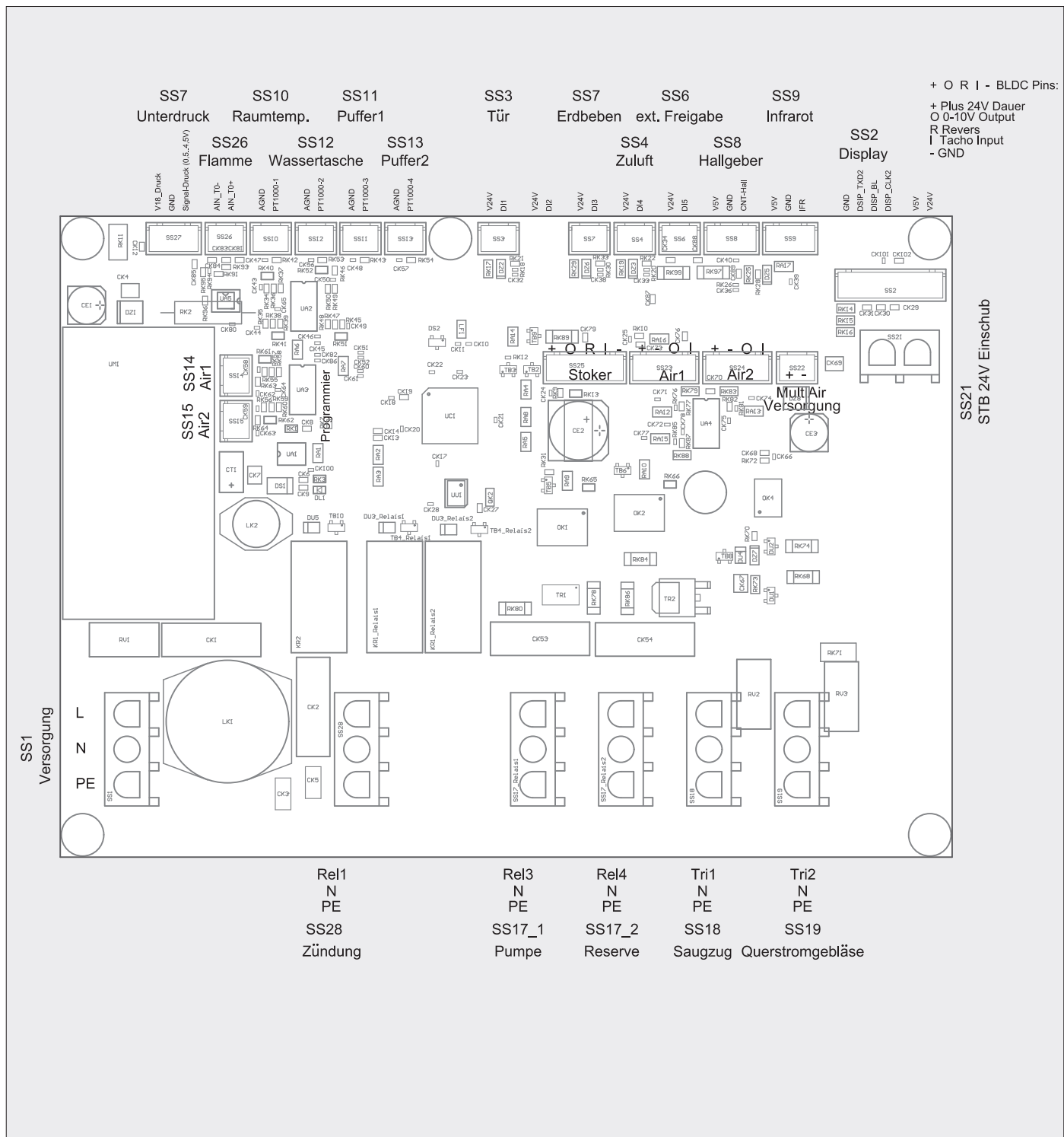
Abb. 2.22 Elektrischer Anschlussplan
