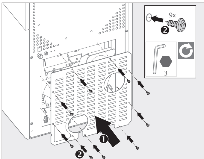
Fig. 2.17 Monter la paroi arrière et le clapet fourni
