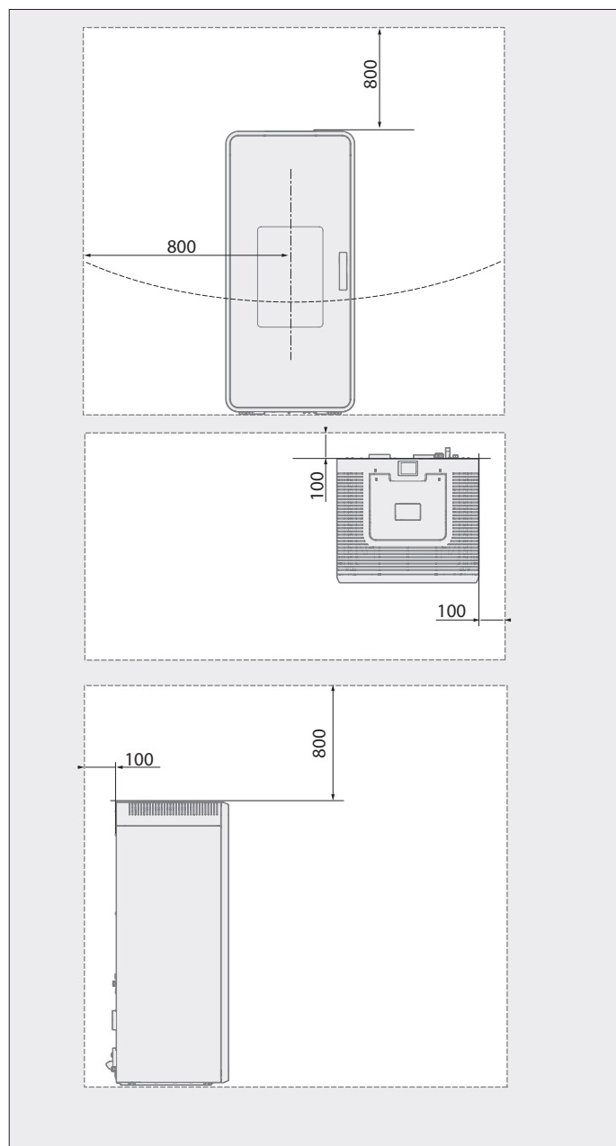
Abb. 2.5 Mindestabstände
