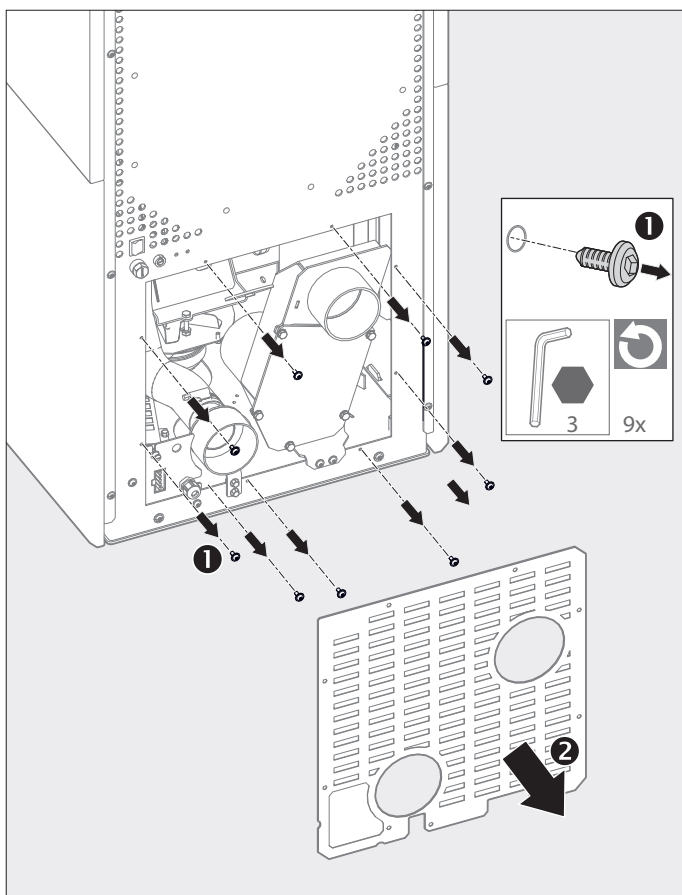
Abb. 2.9 Untere hintere Rückwand und Blende demontieren
