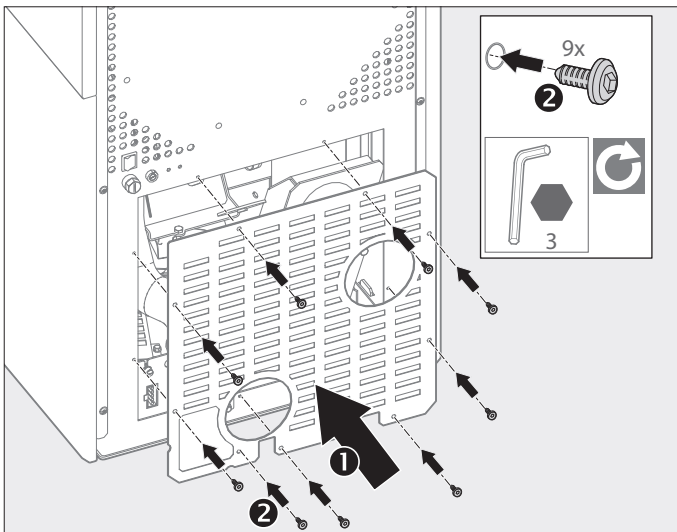
Abb. 2.17 Untere Rückwand montieren
