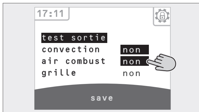
Fig. 2.19 Vérification du fonctionnement dans le menu Test relais
