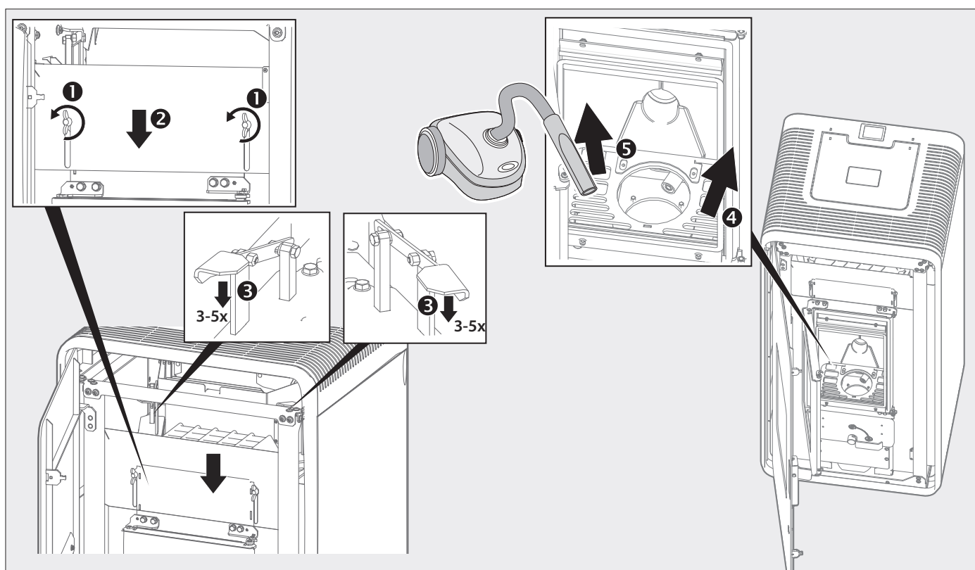
Abb. 4.2 Nettoyer le foyer – actionnement des curseurs de nettoyage
