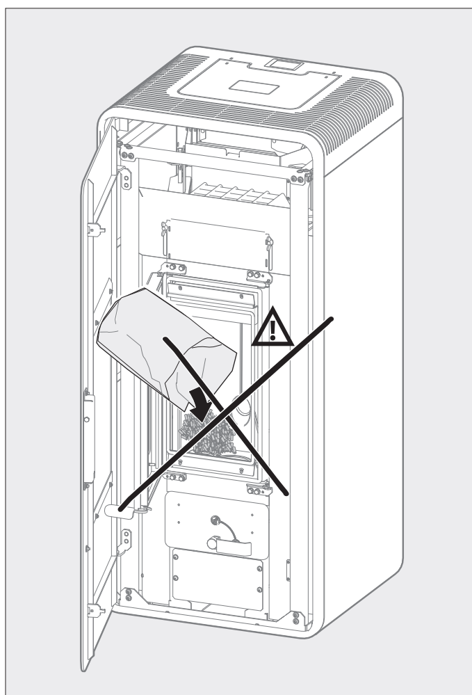
Fig. 3.7 Ne pas placer de granulés manuellement dans la cuvette de combustion, hormis si le réservoir est vide
