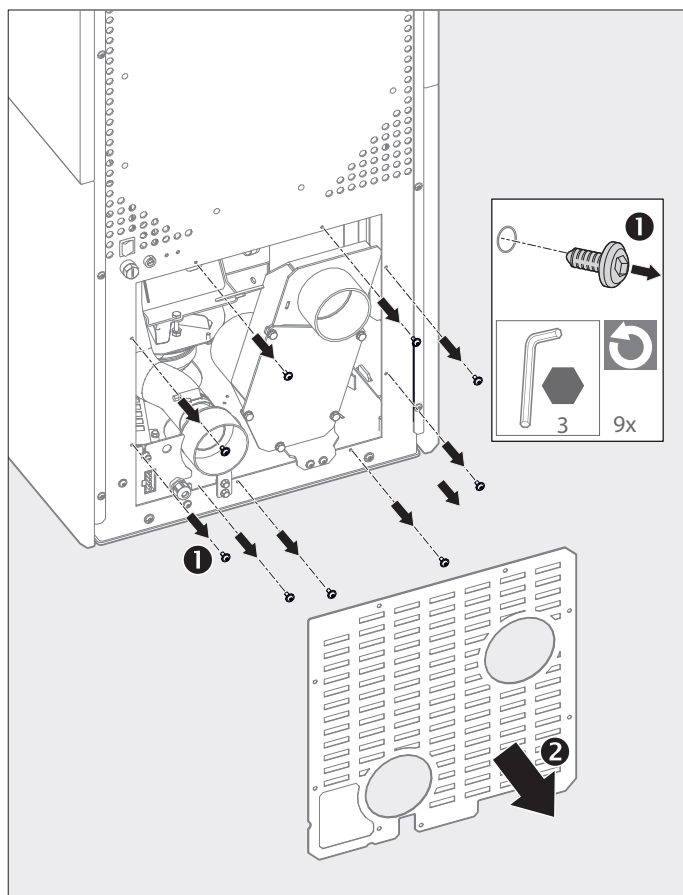
Fig. 2.14 Démontez la paroi
