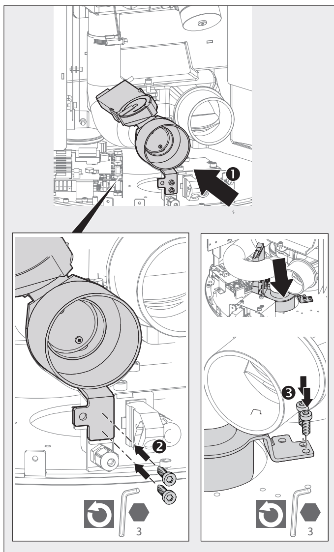
Fig. 2.16 Monter la paroi arrière et le clapet fourni
