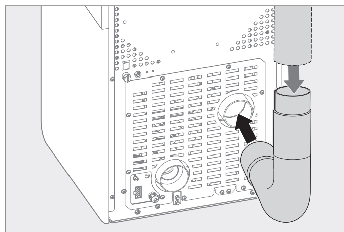
Fig. 2.7 Placer la tubulure d'échappement sur le raccord (sur site)
