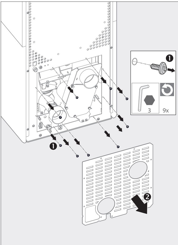
Abb. 2.14 Untere Rückwand demontieren
