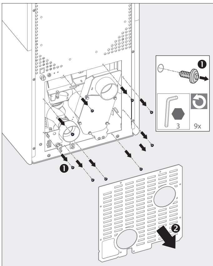
Fig. 2.9 Démontez la paroi arrière et le clapet
