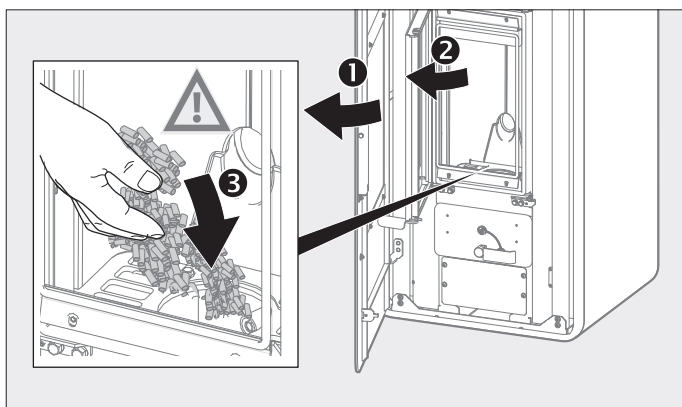
Fig. 2.22 Remplissage manuel des granulés lors que le puits à granulés est vide
