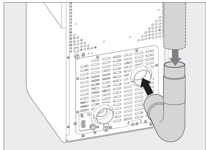
Abb. 2.7 Abgasrohr (bauseitig) auf Anschlussstutzen stecken
