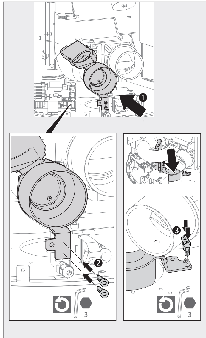
Abb. 2.16 Motorgesteuerte Verbrennungsluftklappe montieren
