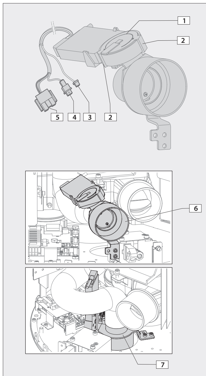
Fig. 2.13 Raccordement d'un clapet d'air de combustion motorisé
