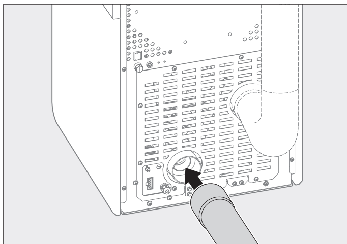
Fig. 2.8 Encastrer la conduite d'air de combustion de Ø 80 mm à l'arrière
