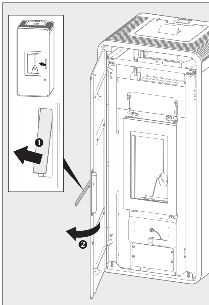
Abb. 3.10 Tür öffnen und schließen
