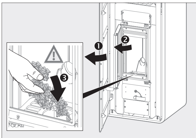
Abb. 2.23 Pellets bei leerem Pelletschacht mit der Hand einfüllen
