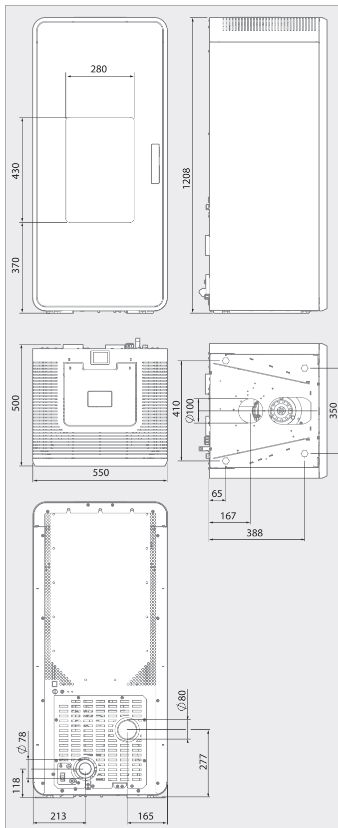
Fig. 2.4 Dimensions
