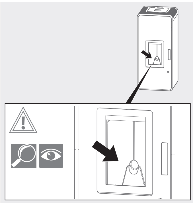
Abb. 3.2 Sichtprüfung Brennermulde
