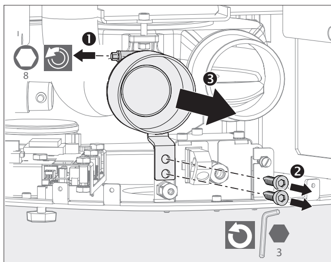
Fig. 2.15 Dévisser le manchon d'arrivée d'air de combustion
