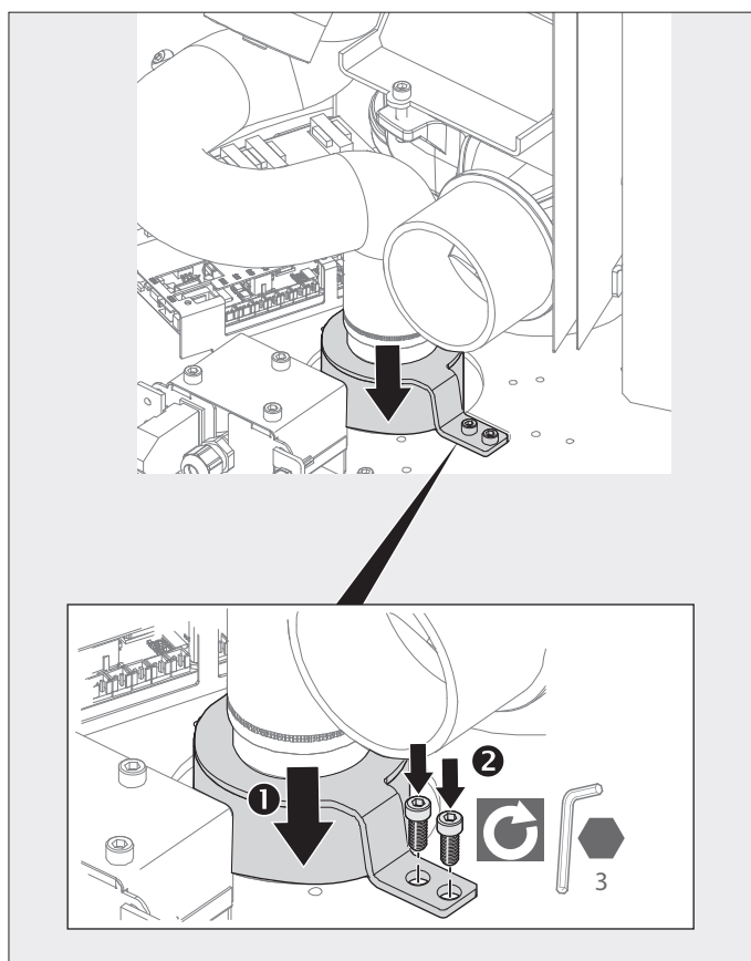
Fig. 2.11 Vissez le manchon d'arrivée d'air de combustion à la tôle de fond
