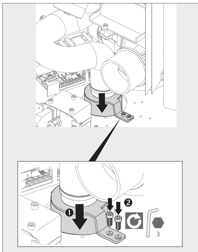
Abb. 2.11 Verbrennungsluftstutzen an Bodenblech anschrauben
