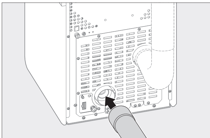
Abb. 2.8 Verbrennungsluftleitung Ø 80 mm hinten aufstecken
