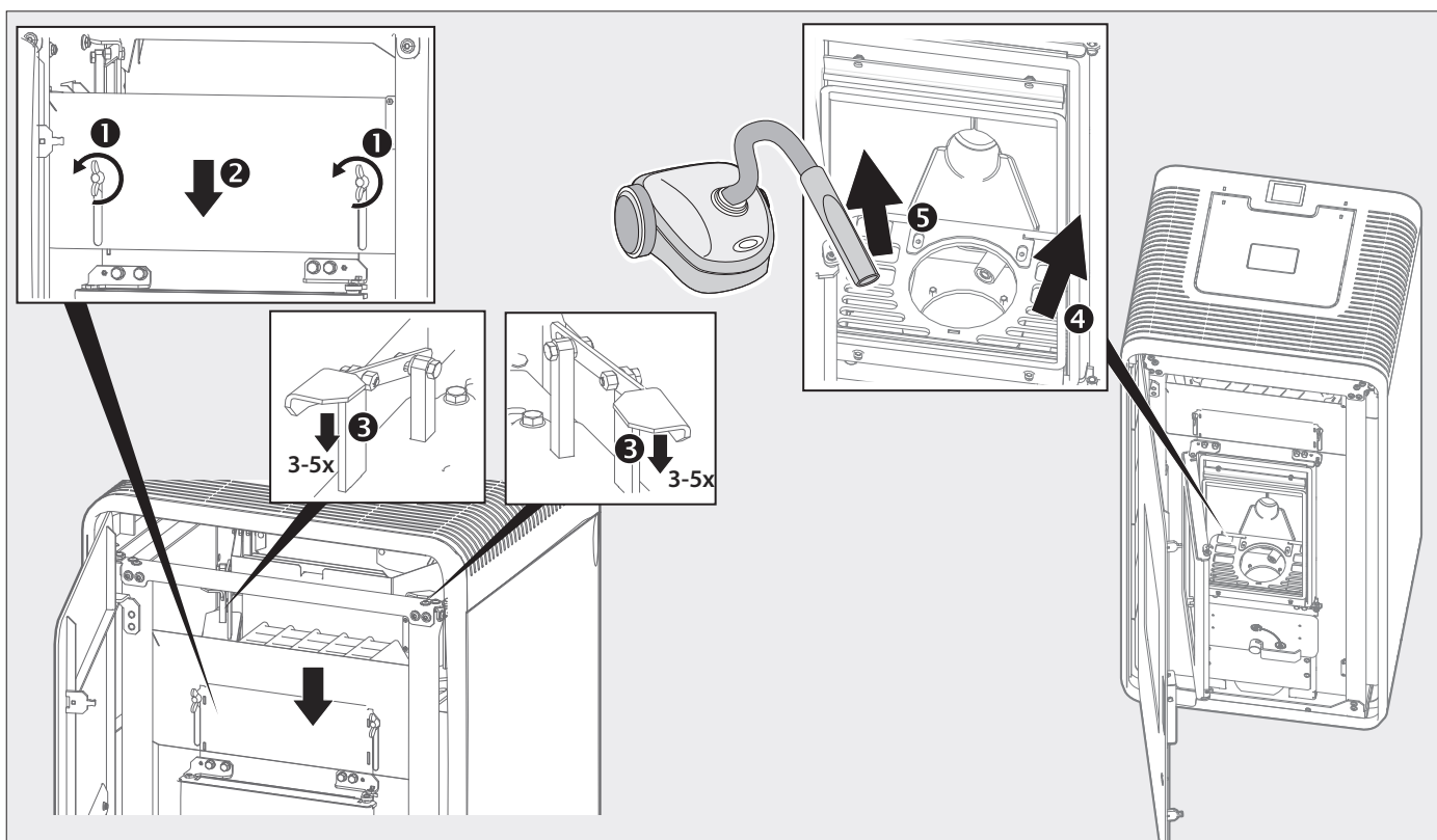
Abb. 4.2 Feuerraum reinigen – Betätigung der Reinigungsschieber
