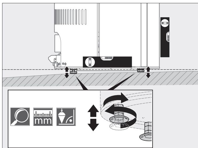
Fig. 2.20 Aligner le poêle à granulés avec les pieds réglables en hauteur
