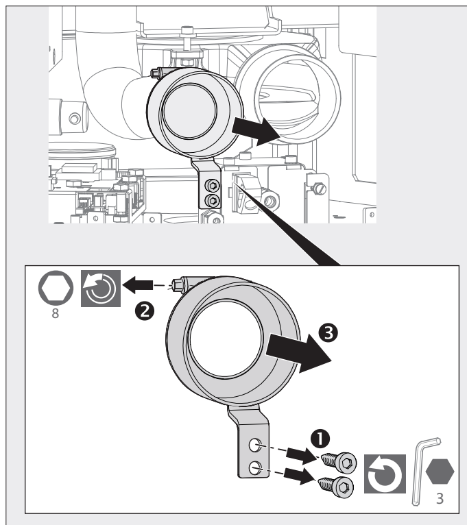
Abb. 2.10 Verbrennungsluftstutzen abschrauben
