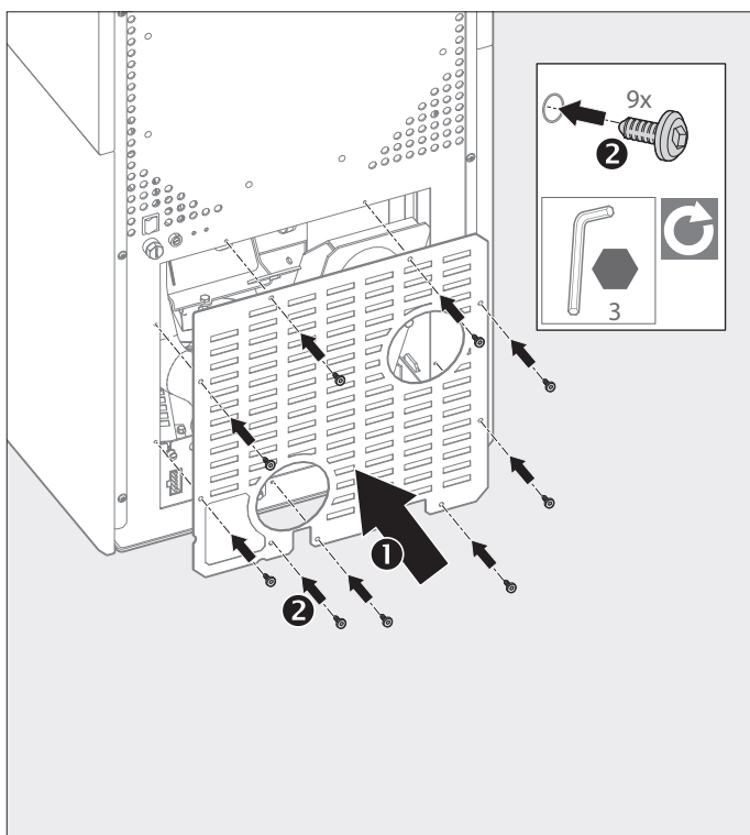
Abb. 2.12 Untere Rückwand montieren
