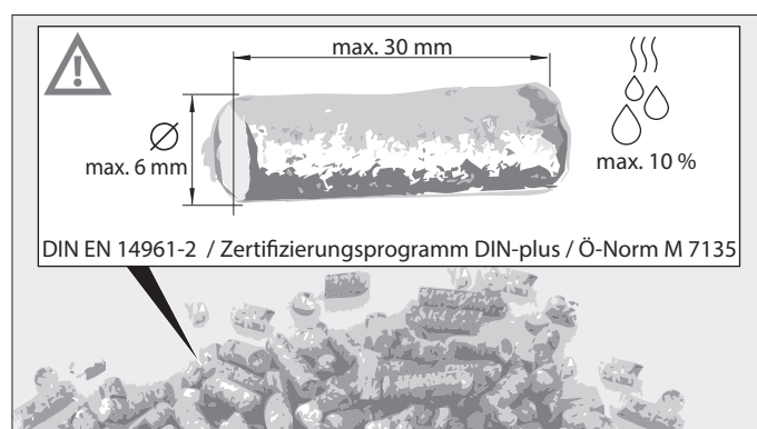
Fig. 3.3 Remplir le réservoir à pellets uniquement avec des granulés autorisés
