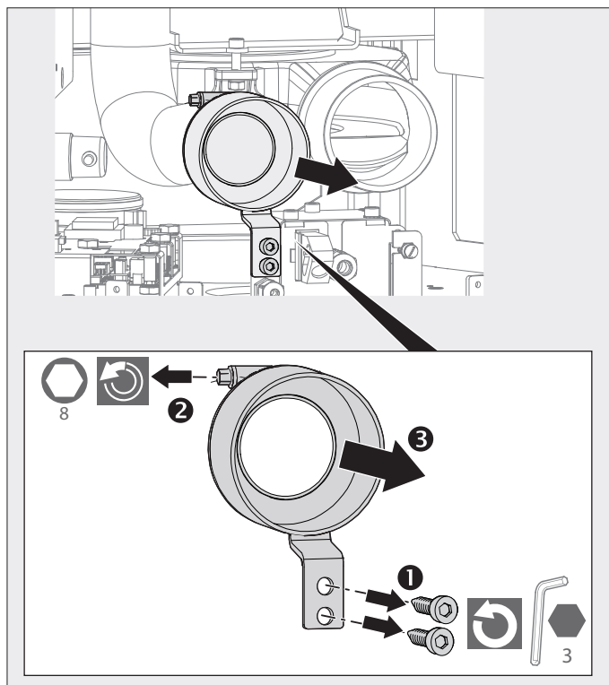
Fig. 2.10 Dévisser le manchon d'arrivée d'air de combustion
