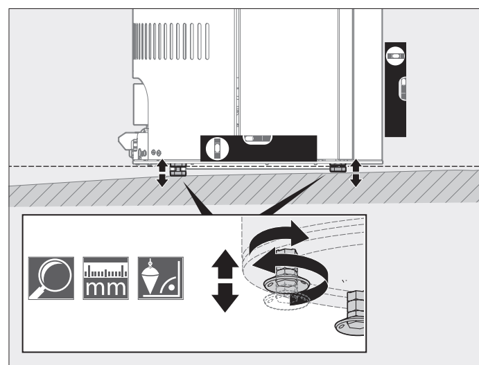
Abb. 2.21 Pellet-Kaminofen mit Stellfüßen ausrichten
