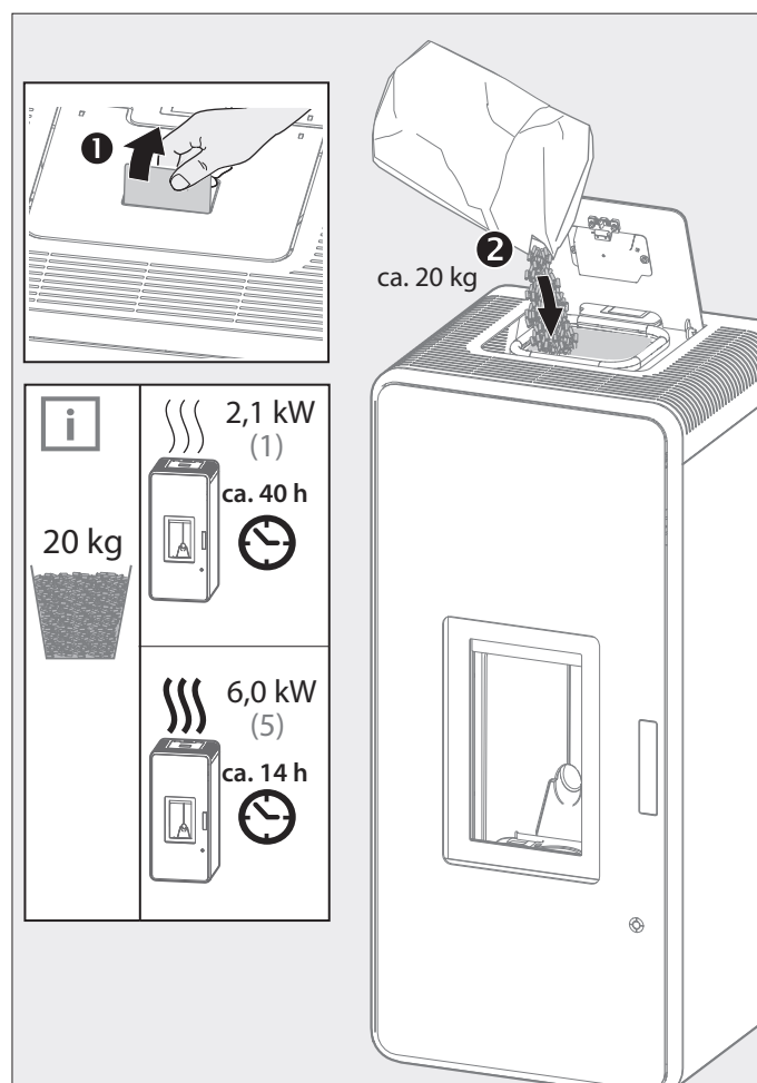
Fig. 3.4 Remplissage des granulés / consommation max./min. de granulés
