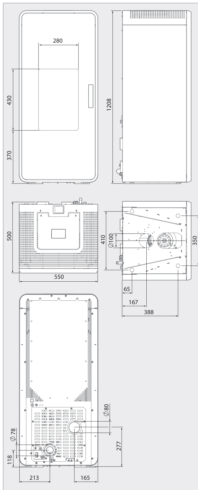
Abb. 2.4 Dimensions
