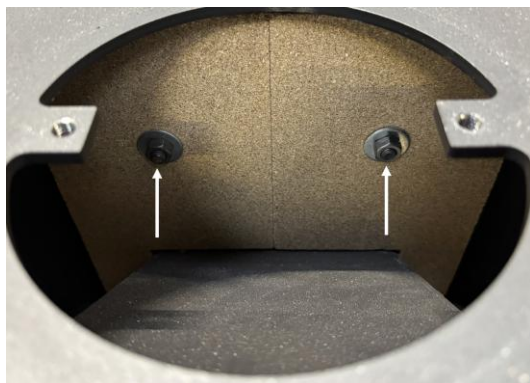
3) Demonteer de 2 moeren aan de binnenkant van de verbrandingskamer.
