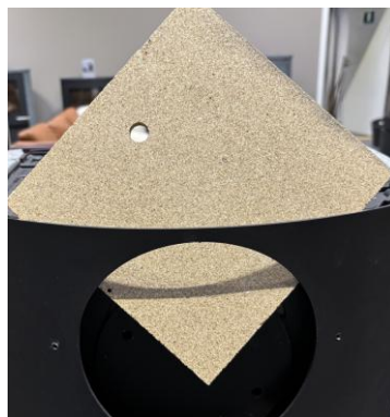
6) Fjern vermiculitt og dekkplate.
