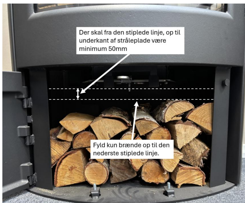
Figur 11 - Brænde opbevaring
