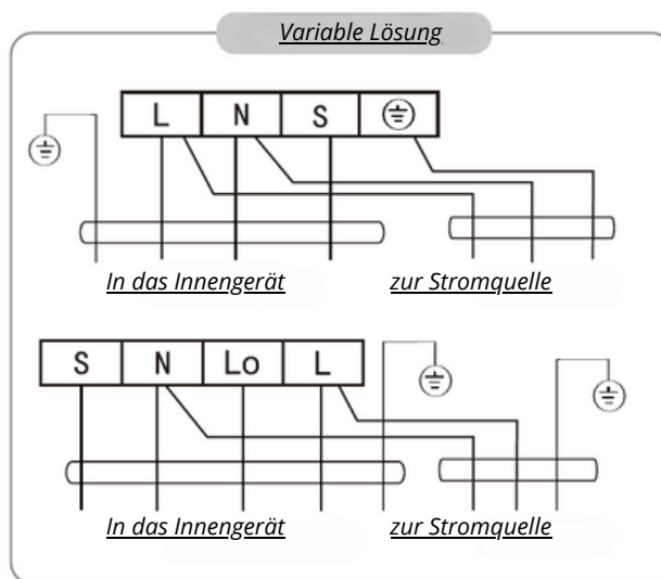
Konnektor
