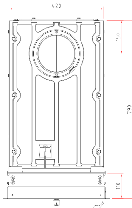
Draufsicht M 1:10
