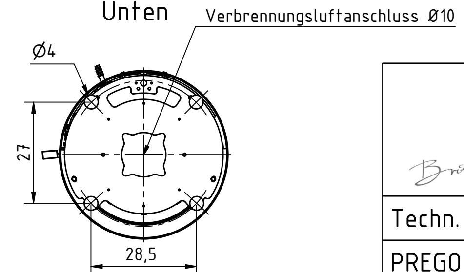
Verbrennungsluftanschluss Ø10
